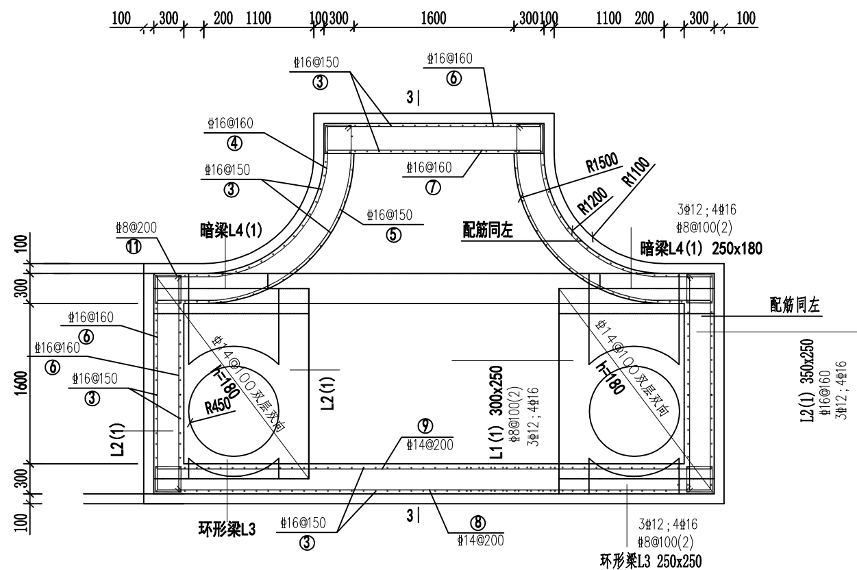
结构平面图 1:50
