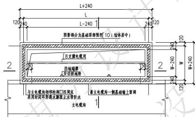
环网箱基础平面图
