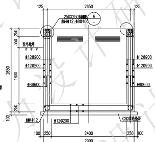
4- -4断面
