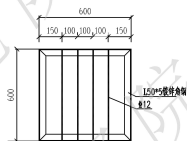
铁篦子
