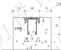
预埋槽钢详图
