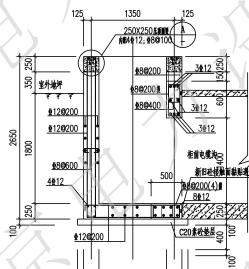
3- -3断面
