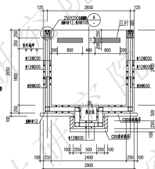
2- -2断面
