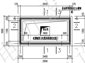
基础平面
