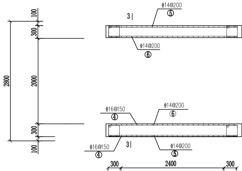
结构平面图 1:50
