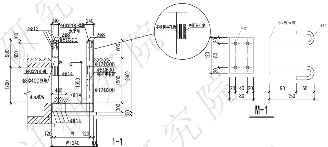
环网箱基础
