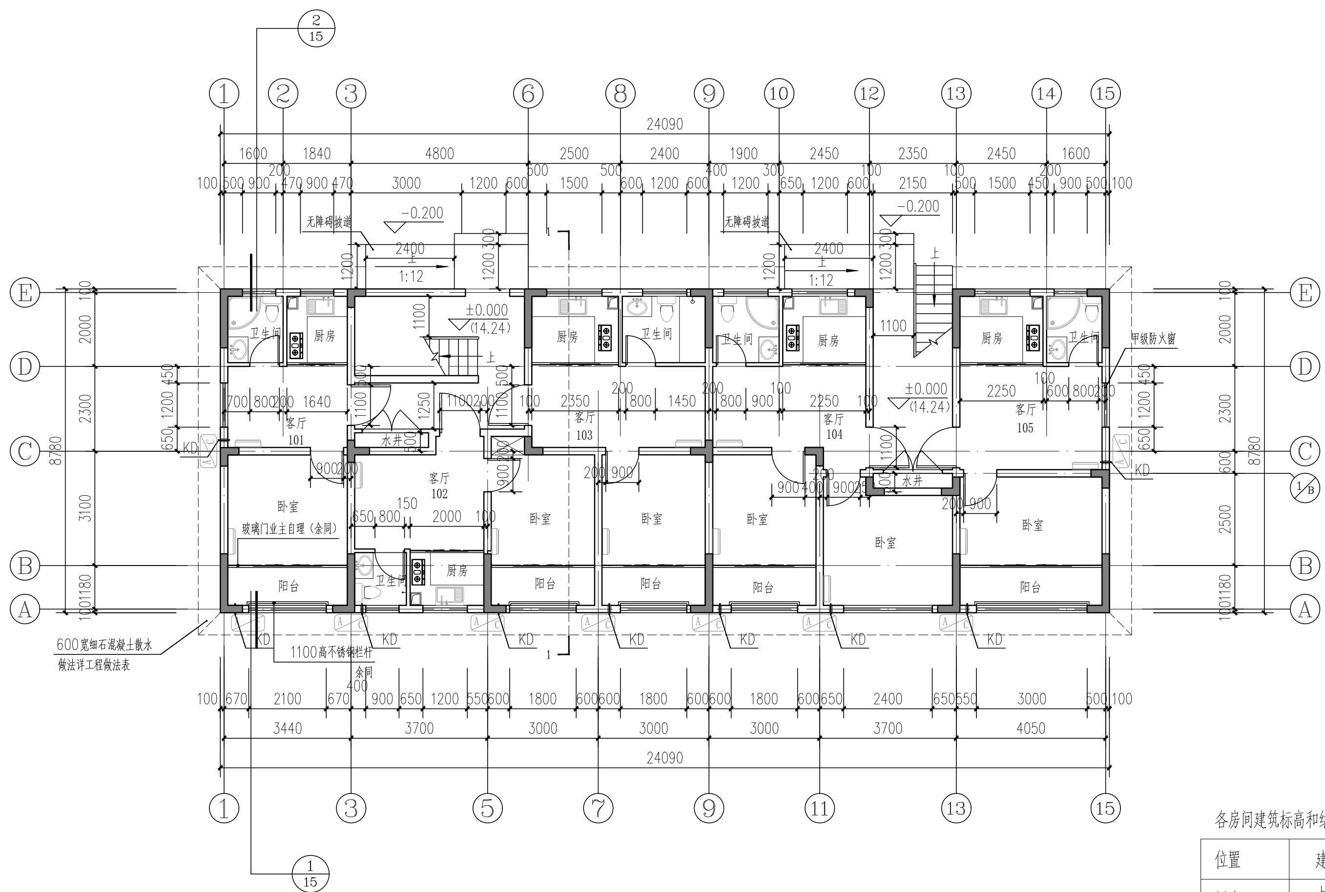
青云巷10-2号 一层平面图 1:100
