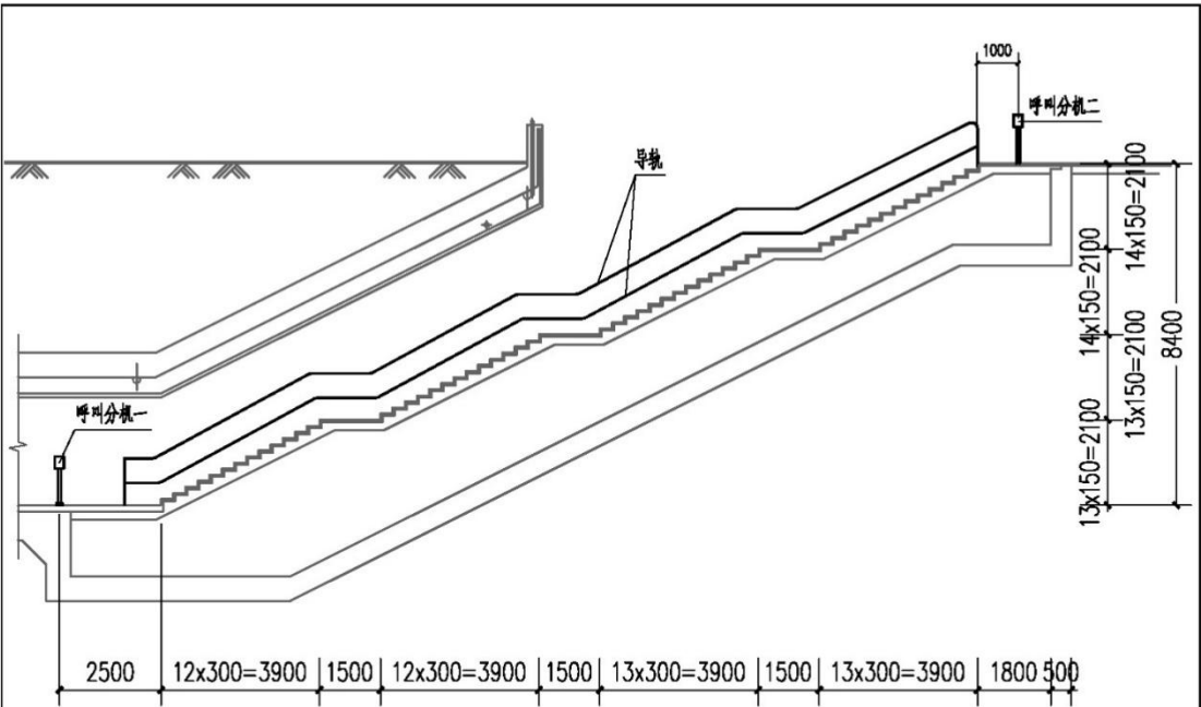
A-A剖面图
