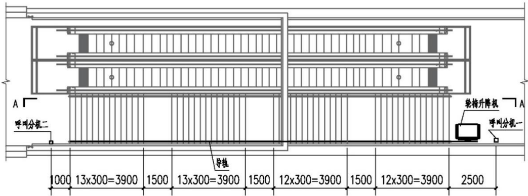
2号出入口轮椅升降机平面布置图
