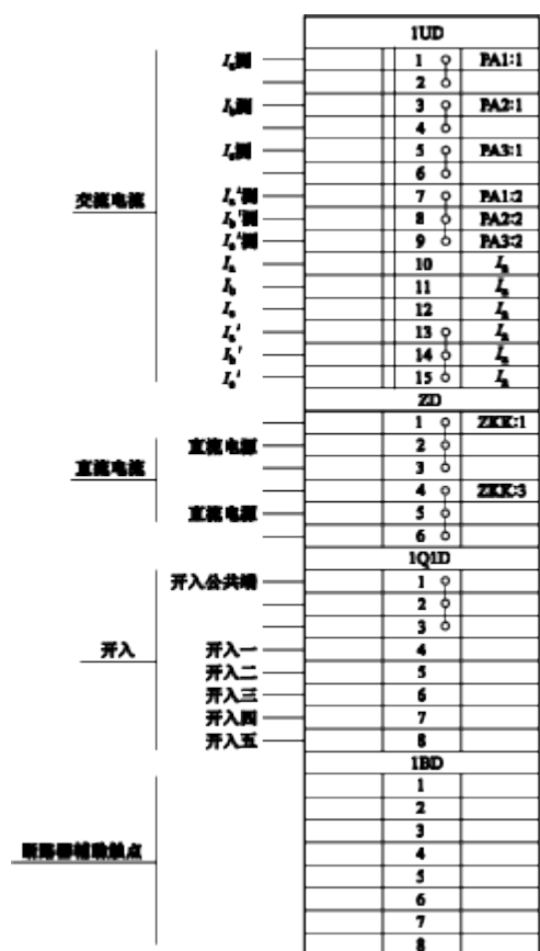
图2 断路器柜端子排图
