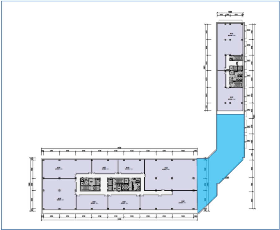
二层屋顶露台设计范围图(蓝色填充区域)
