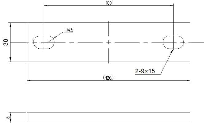
图19 接地排开孔位置示意图
