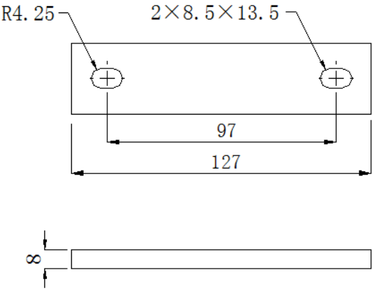
图38 接地排开孔位置示意图
