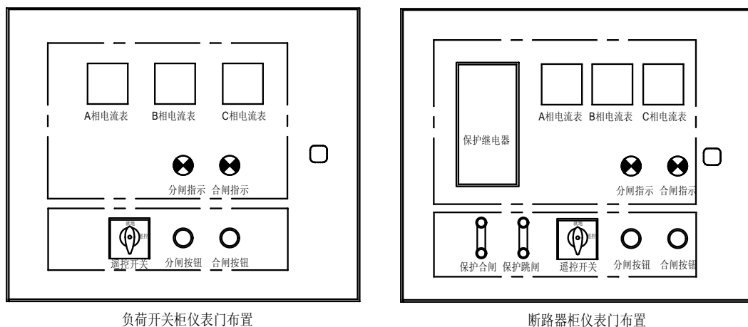
图44 仪表门布置示意图
