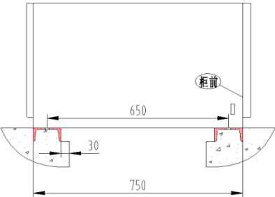
图9 基础槽钢示意图
