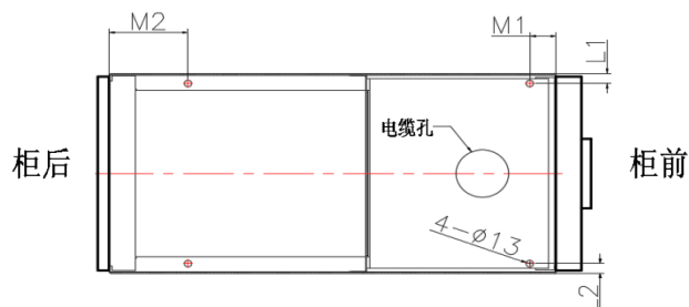
图22 地脚开孔示意图
