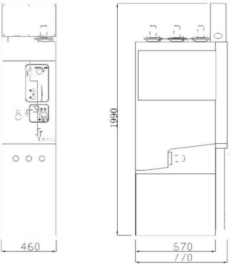
图36 顶扩展外形尺寸图
