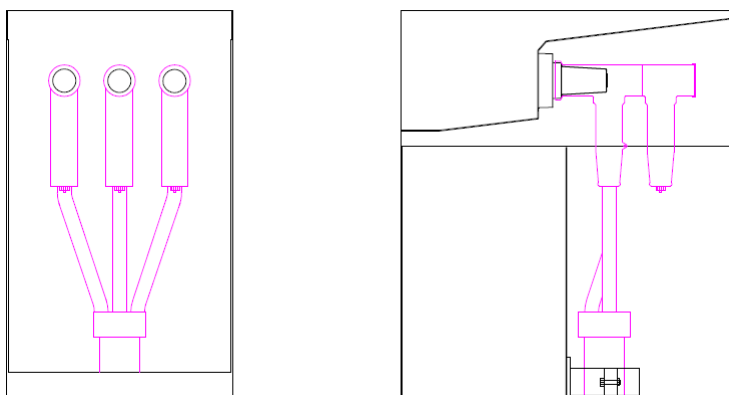
图37 一次电缆固定示意图
