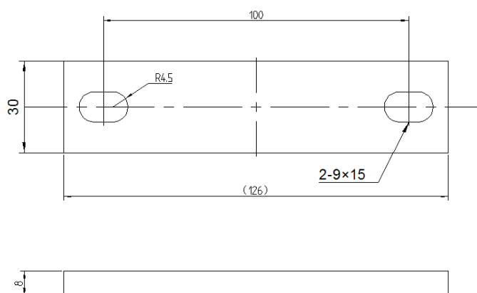
图5 接地排开孔位置示意图
