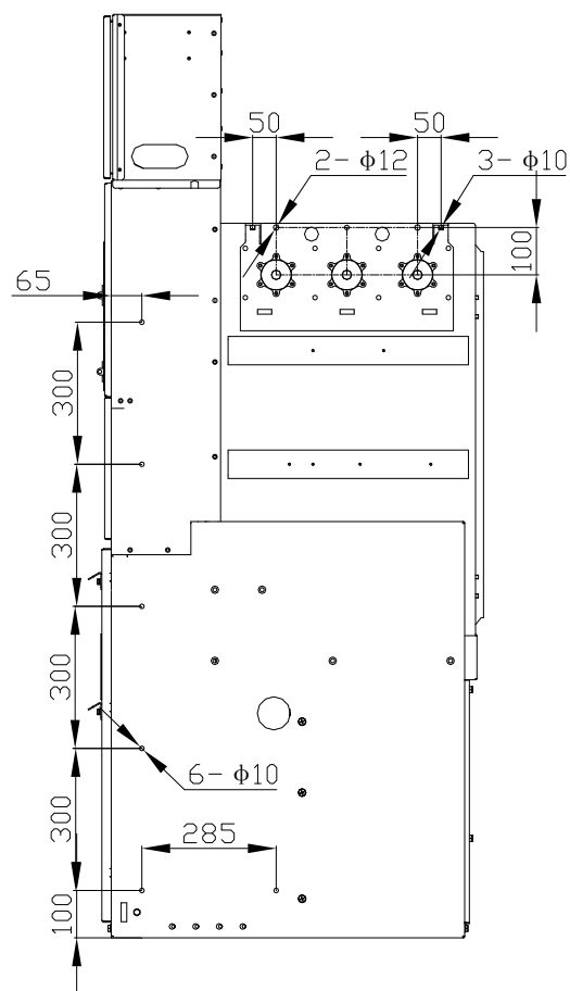
图14 侧出套管并柜孔位置示意图
