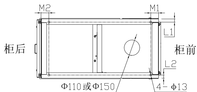
图8 地脚开孔位置示意图
