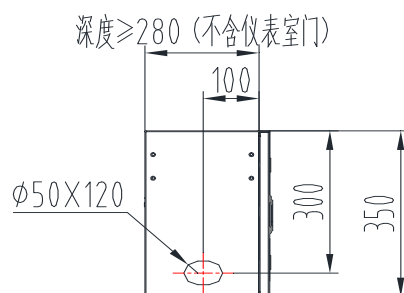
图32 二次仪表室接口尺寸图
