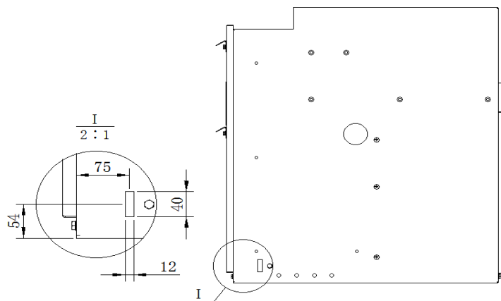
图6 一次接地排在柜体贯穿孔尺寸及位置示意图
