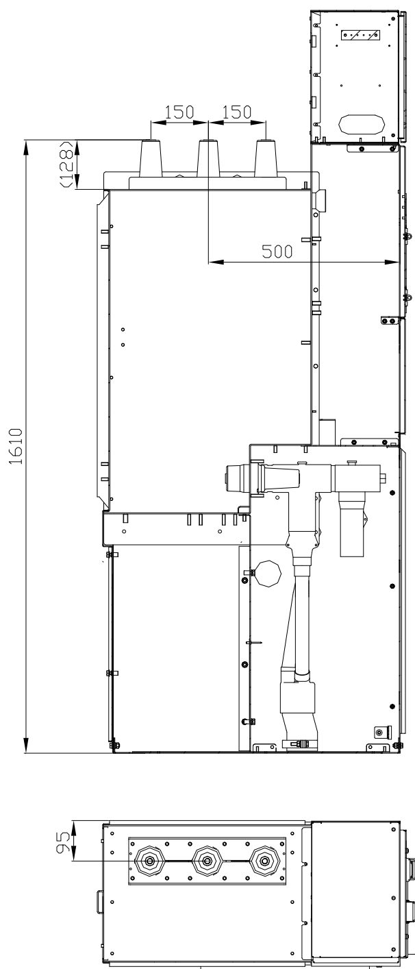
图15 上出套管位置示意图
