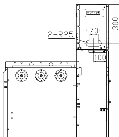
图21 仪表箱二次走线孔示意图
