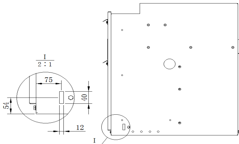
图20 一次接地排在柜体贯穿孔尺寸及位置示意图
