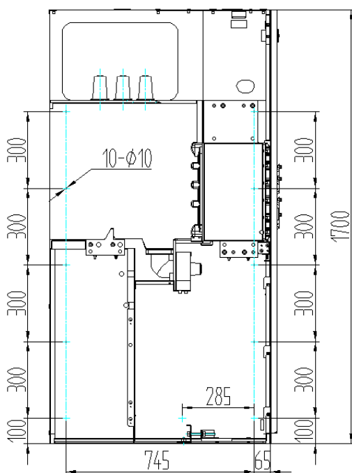
图31 各柜型方案2并柜孔分布尺寸图
