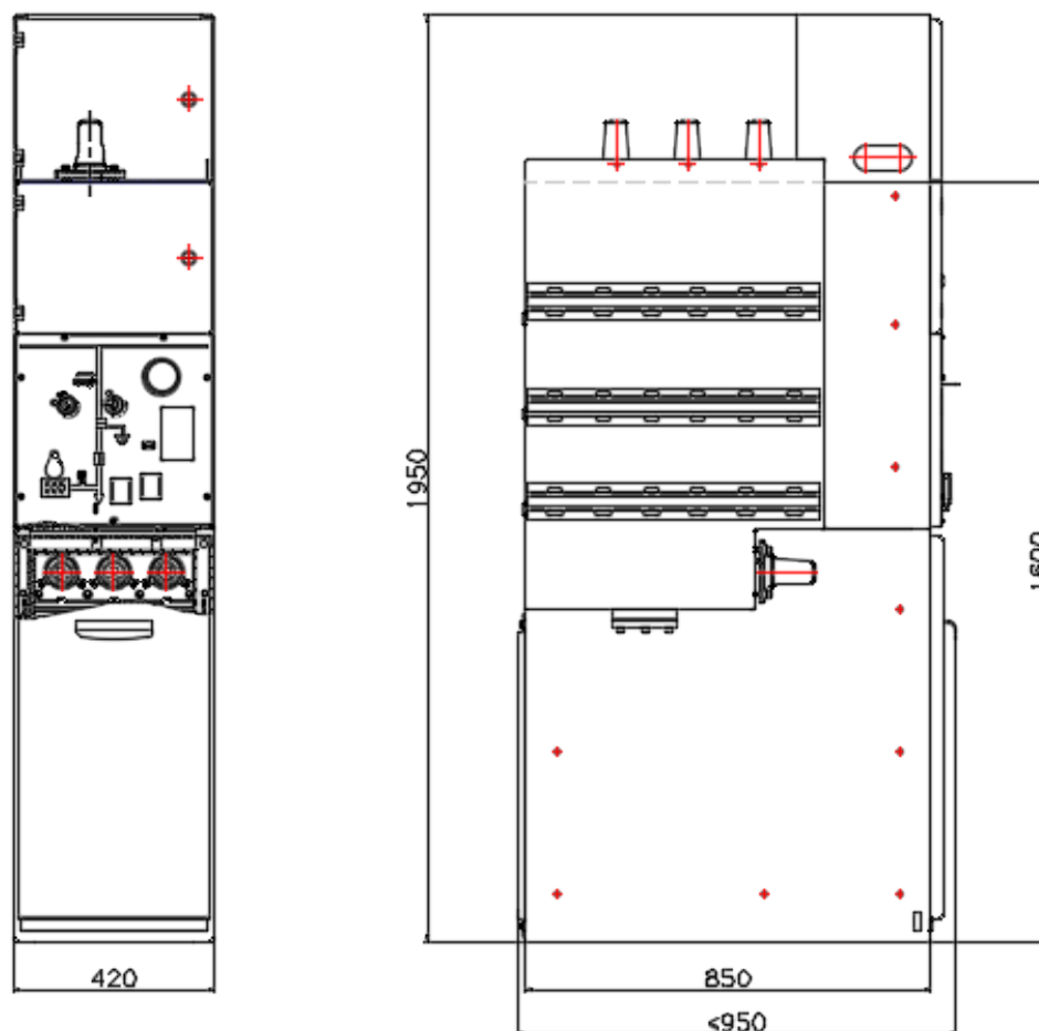
图18 顶扩柜体外形尺寸图
