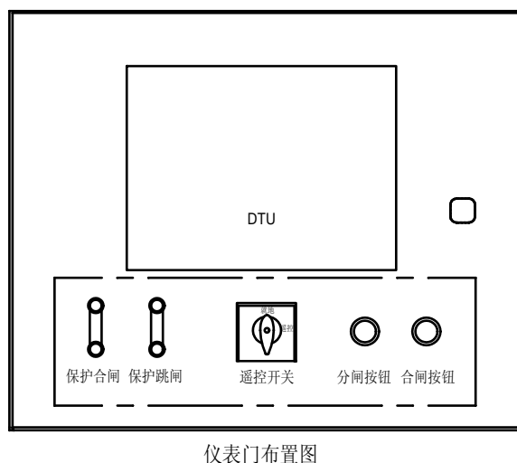
图45 仪表门安装分布式DTU布置示意图
