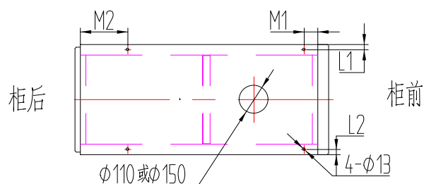
图33 地脚开孔位置示意图
