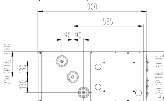
图27 各柜型定制方案2母线套管位置尺寸图（柜体俯视图）
