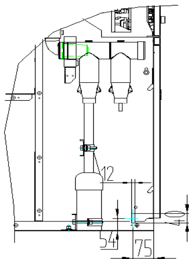
图29 一次接地排位置尺寸图
