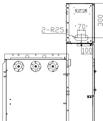
图7 仪表箱二次走线孔示意图
