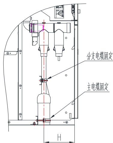
图25 一次电缆固定位置示意图
