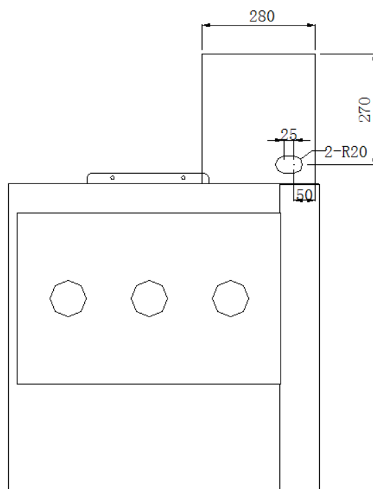
图40 仪表箱二次走线孔示意图
