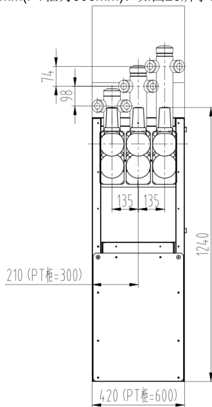
图26 各柜型定制方案1母线套管位置尺寸图（柜体后视图）
