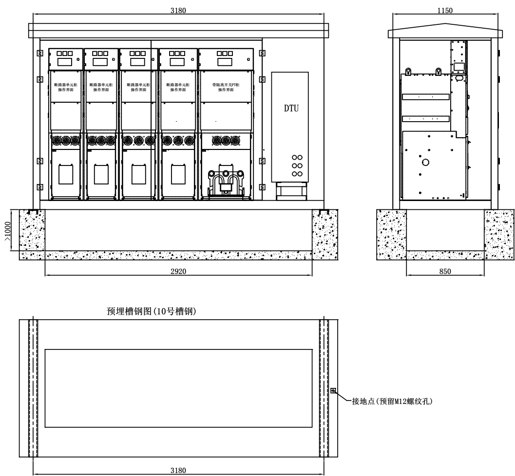
图48 户外环网箱（VVV）地基接口尺寸图
