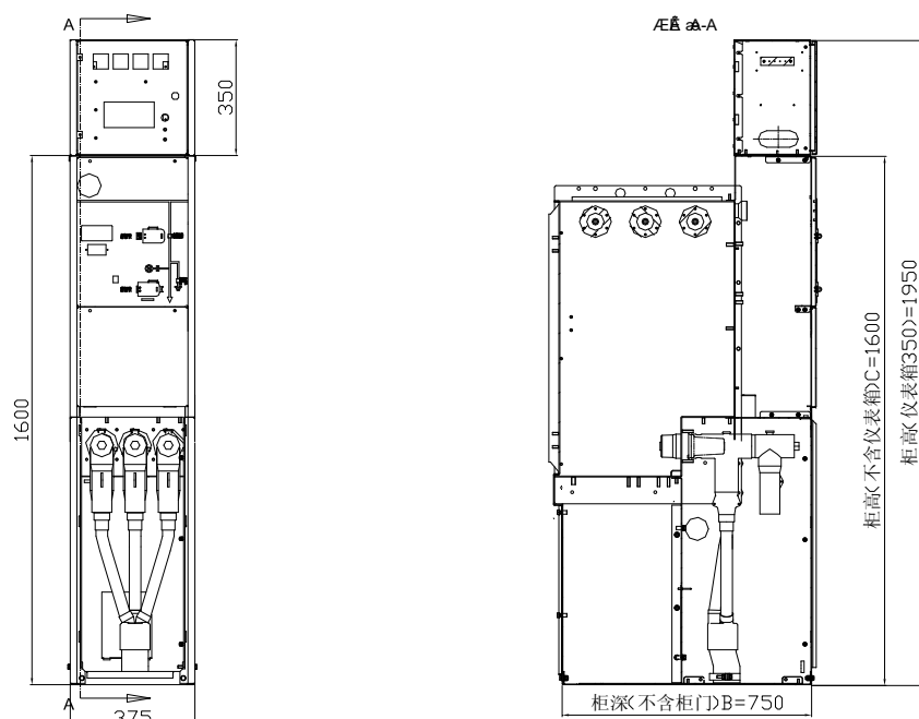
图2 柜高示意图
