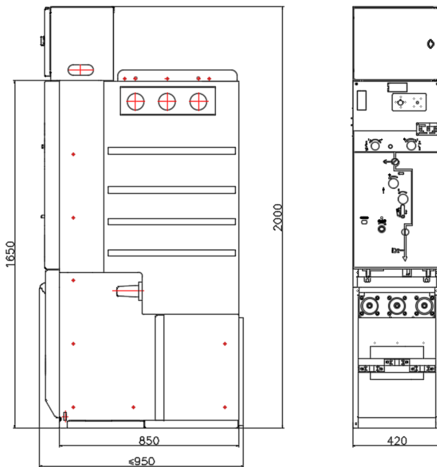
图17 侧扩柜体外形尺寸图
