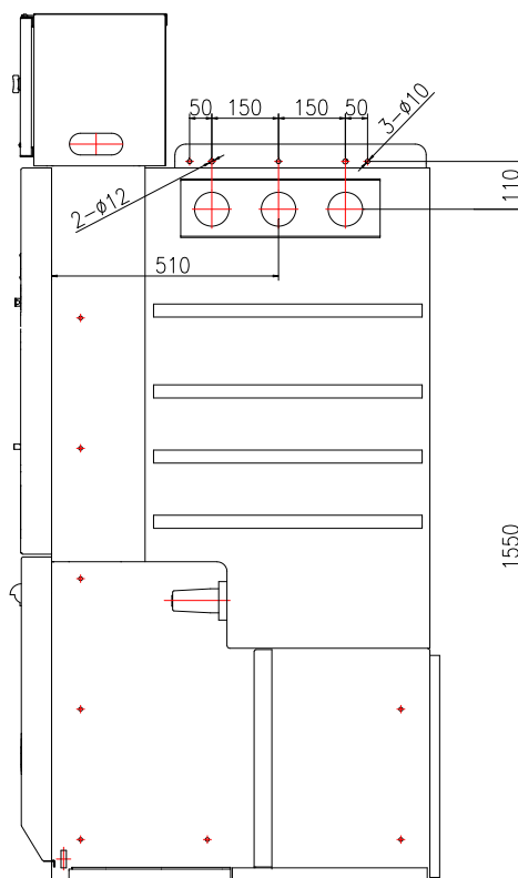
图23 侧扩并柜尺寸图
