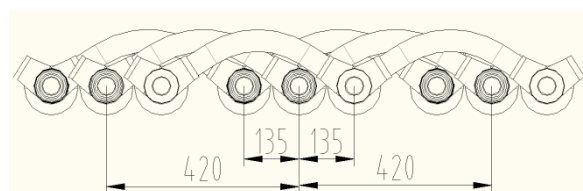
图28 母线连接尺寸图
