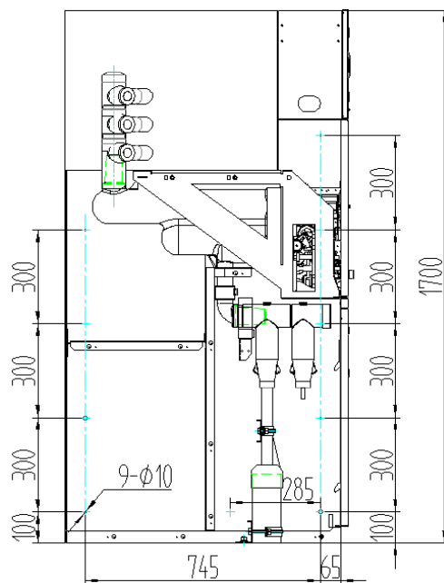
图30 各柜型定制方案1并柜孔分布尺寸图
