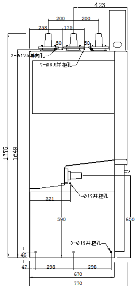
图43 顶扩并柜尺寸图
