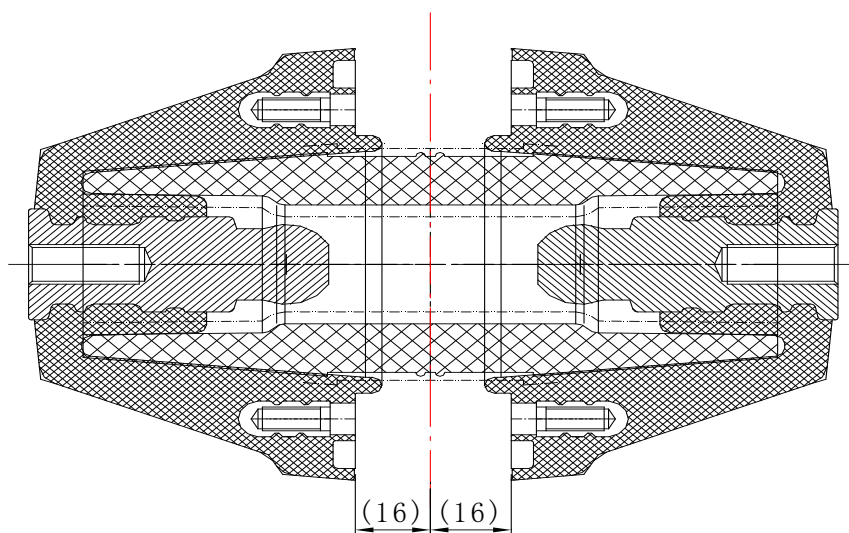
图13 母线插座与连接器并柜尺寸示意图
