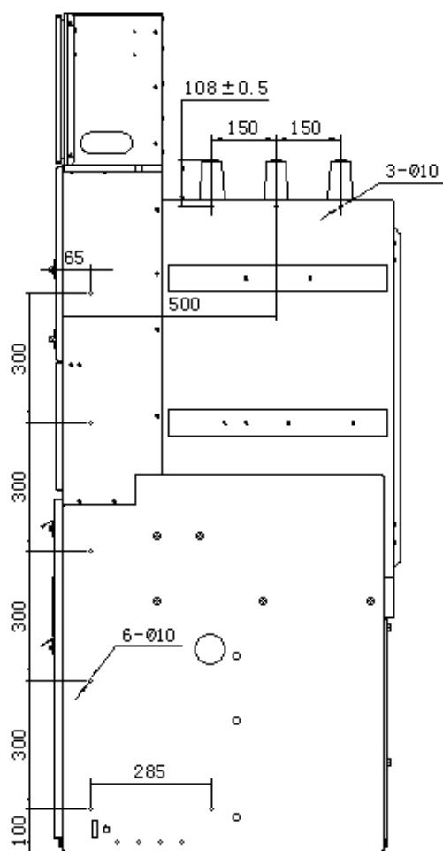
图16 顶出套管并柜孔位置示意图
