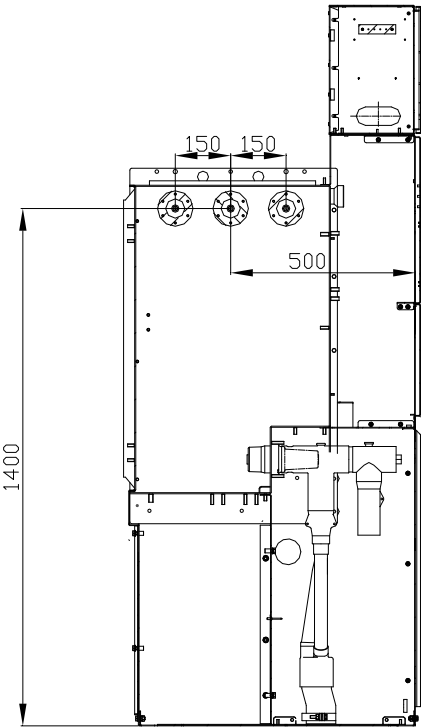
图10 侧出套管位置示意图
