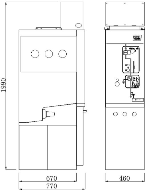
图35 侧扩展外形尺寸图
