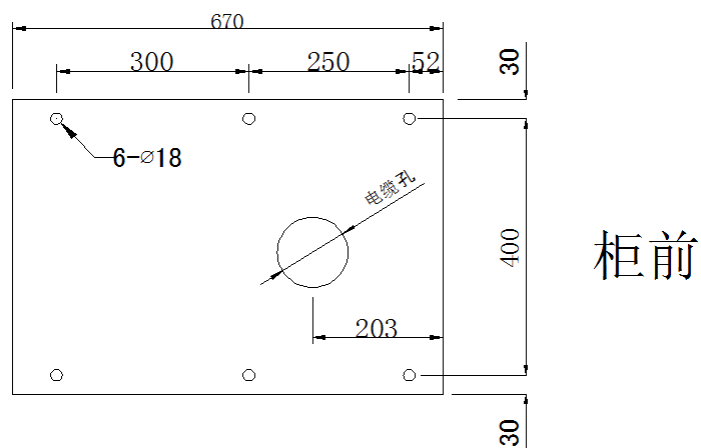
图41 地脚开孔示意图
