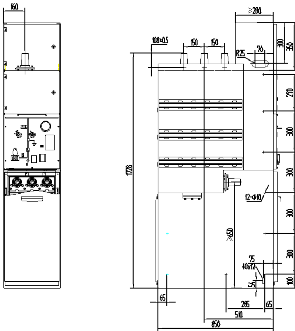
图24 顶扩并柜尺寸图
