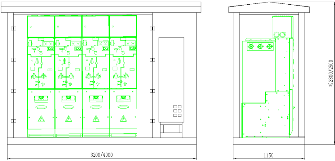
图47 环网箱外形尺寸图
