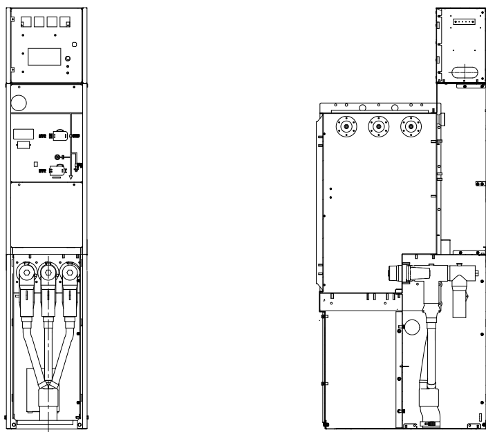
图4 一次电缆孔位置示意图
