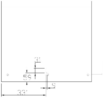
图39 一次接地排在柜体贯穿孔尺寸及位置示意图
