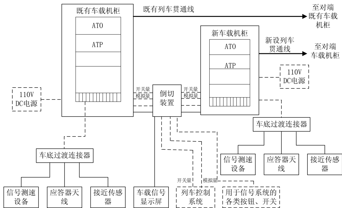
图 2.1-1 车辆与信号系统供货范围示意图
