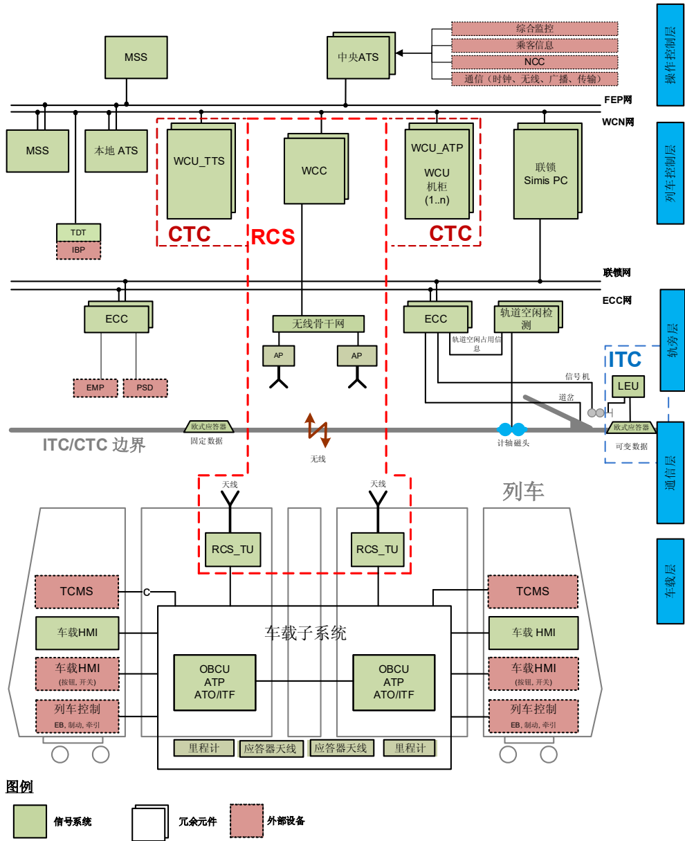
图 3.1-1 信号系统结构示意图
