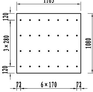
N4钢板
