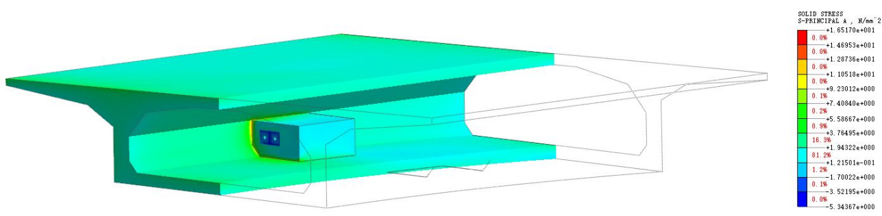
图 6-11 典型齿板有限元分析
