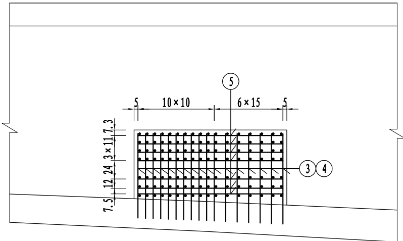
平面
