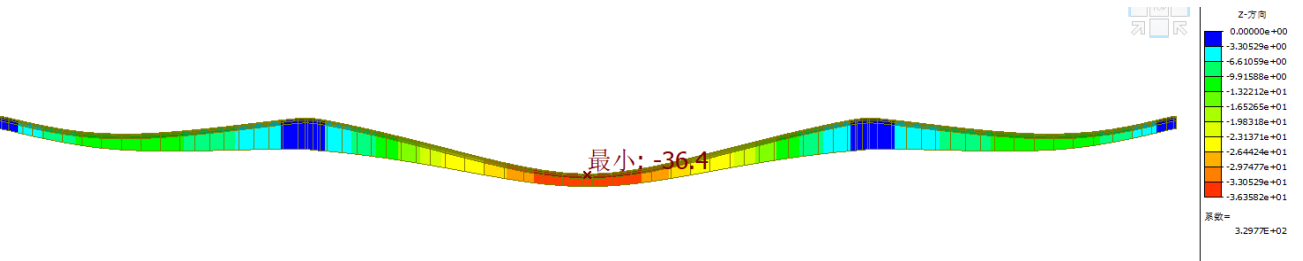
图 6-9 主梁车道荷载竖向挠度图（mm）
