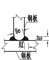
钢板连接大样1
