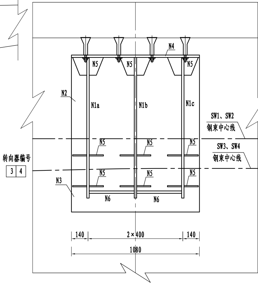
新增转向块2立面图
