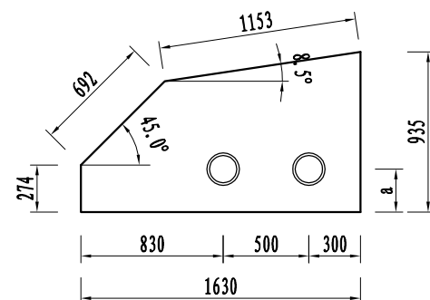
N3钢板
