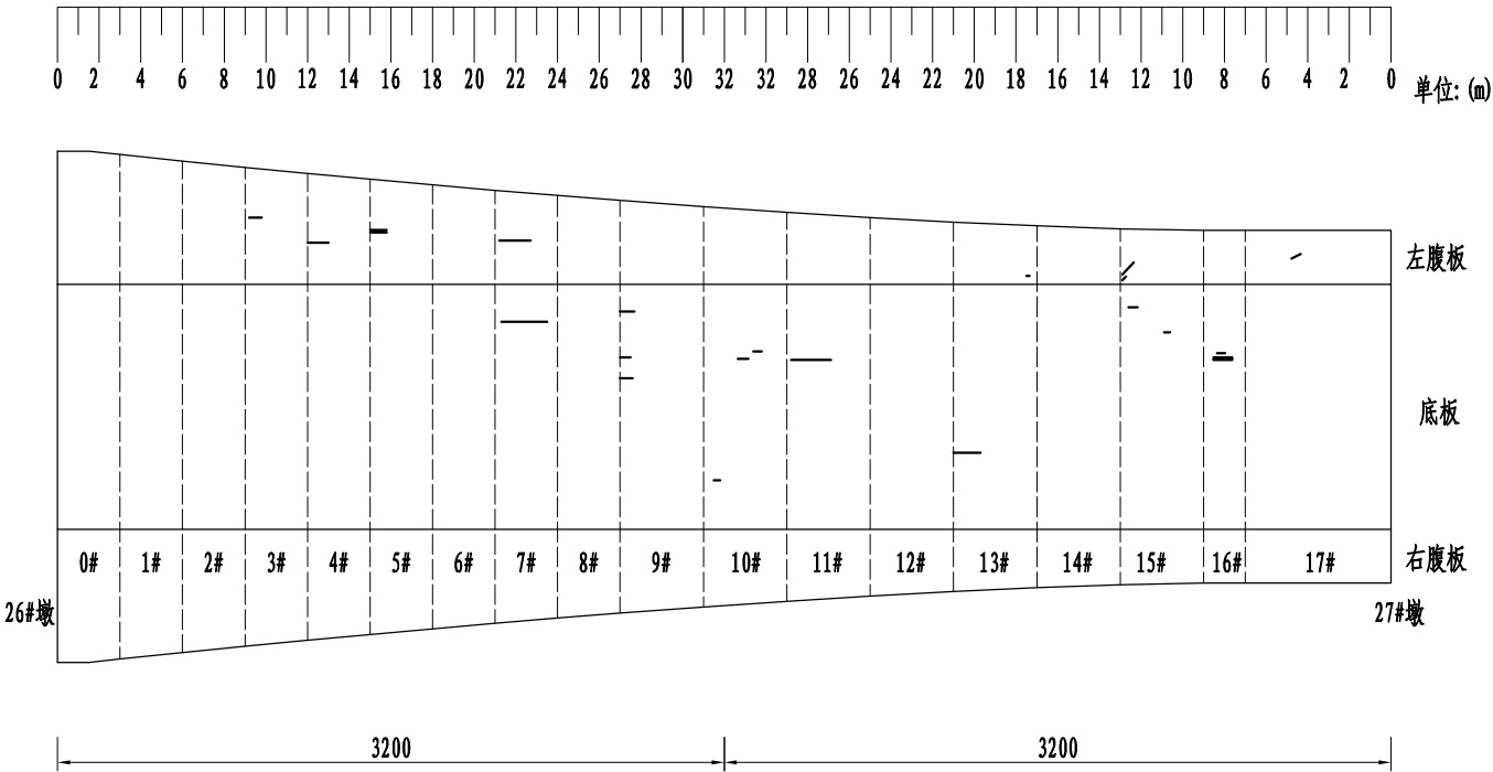
右幅53#孔箱梁外表面病害分布图
