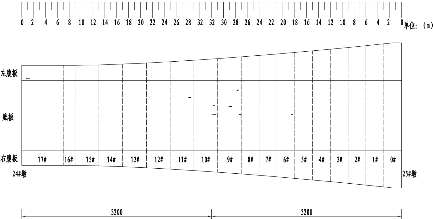
左幅51#孔箱梁外表面病害分布图
