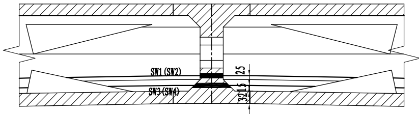
跨中横隔板开孔位置立面示意图
