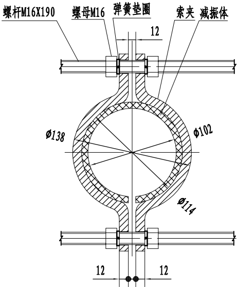
体外预应力钢束减震定位装置示意
