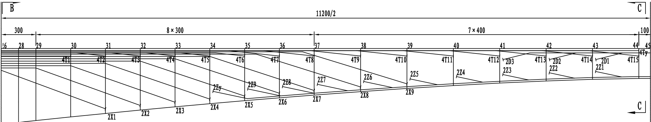
1/2中跨钢束顶板半平面布置
