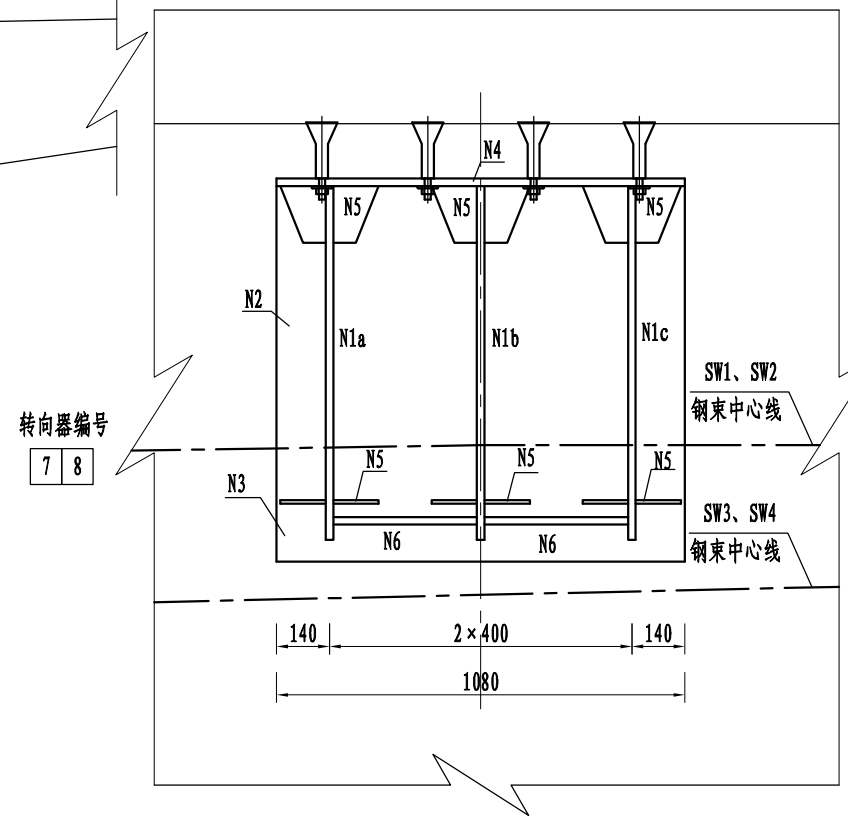
新增转向块4立面图
