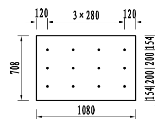
N2钢板
