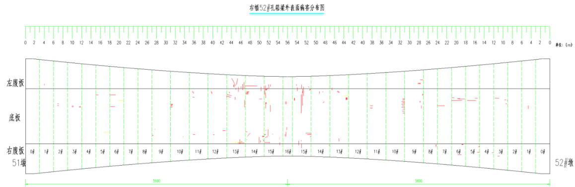
(a) 箱外病害分布图
