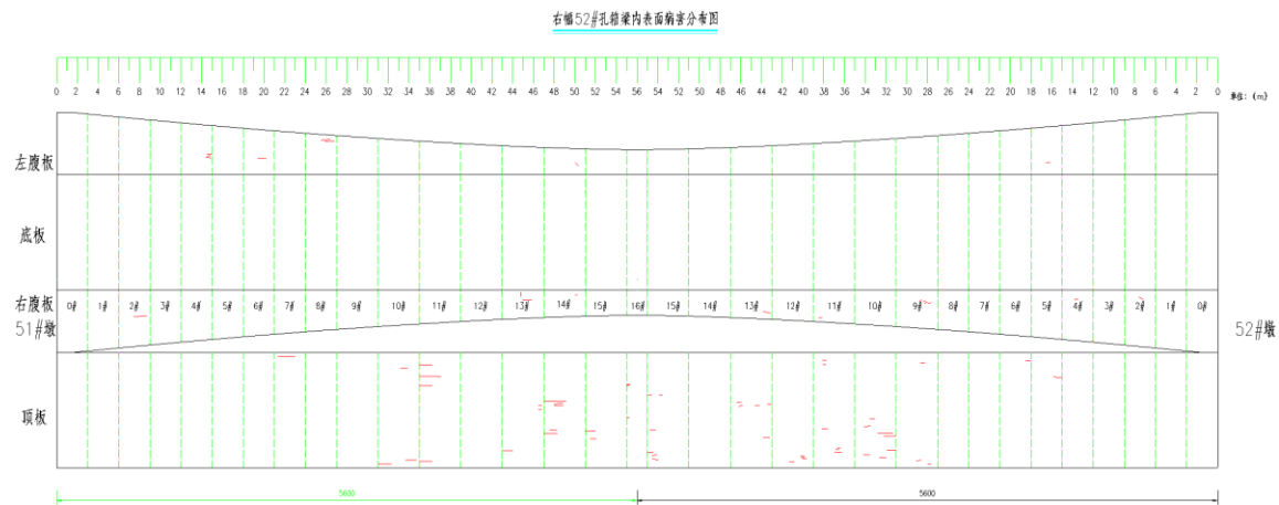
(b) 箱内病害分布图
