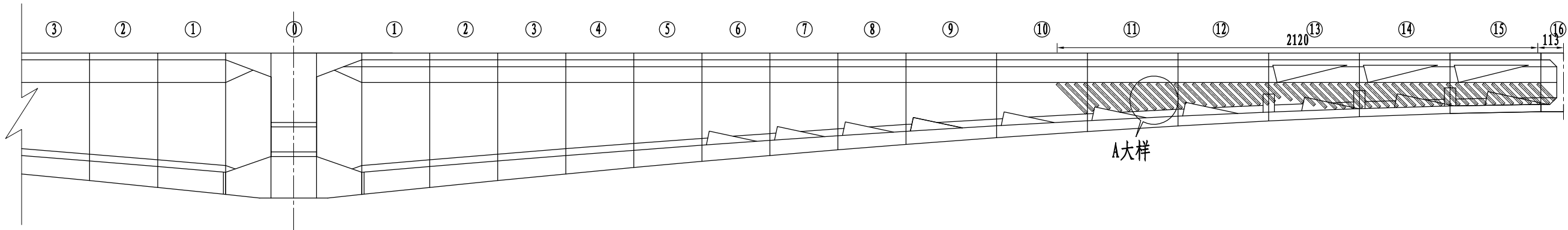
1/2中跨腹板粘贴钢板立面图
