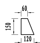
N5钢板
