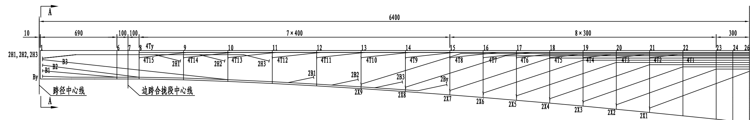
边跨钢束顶板半平面布置
