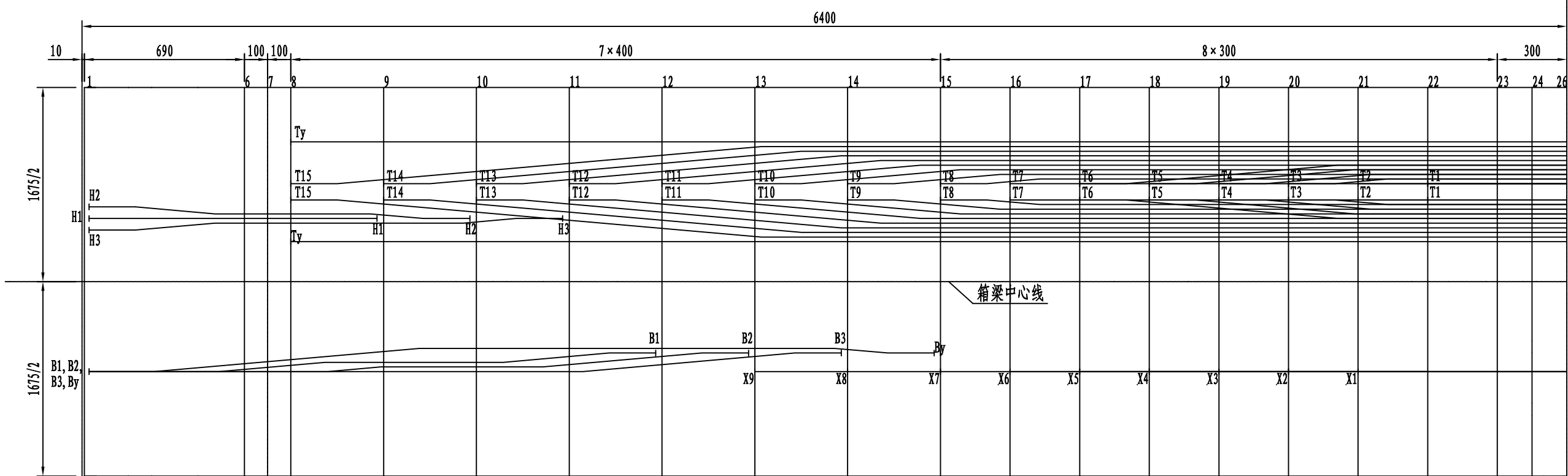
边跨钢束底板半平面布置
