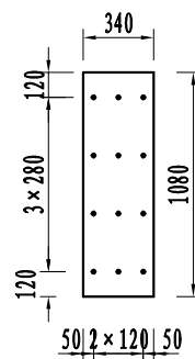
N3钢板
