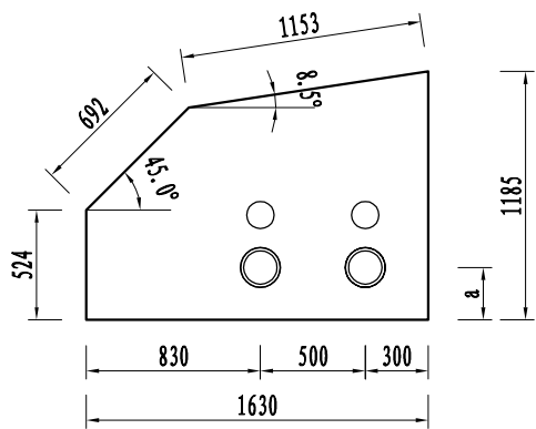
N3钢板
