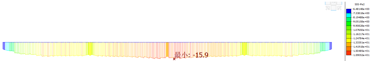
图 6-8 持久状况正常使用极限状态主梁主压正应力包络图（MPa）
