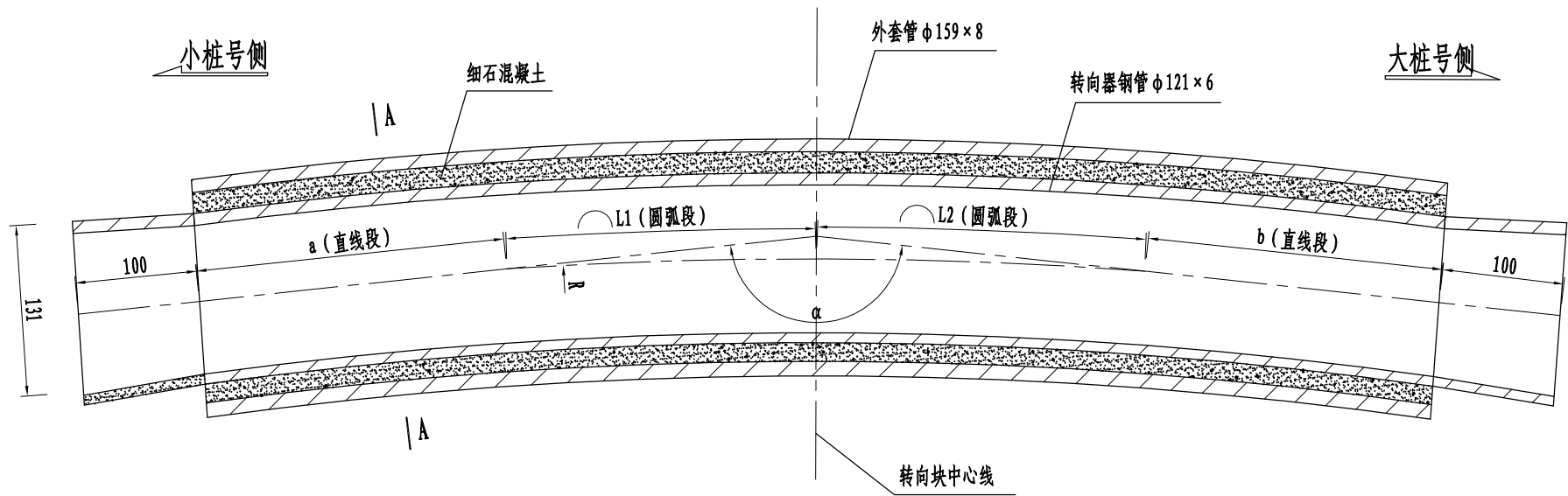
集束式转向器纵断面
