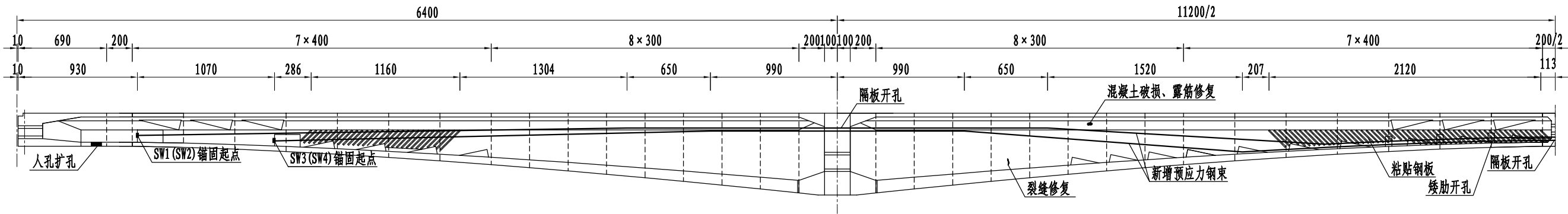
维修加固总体布置图
