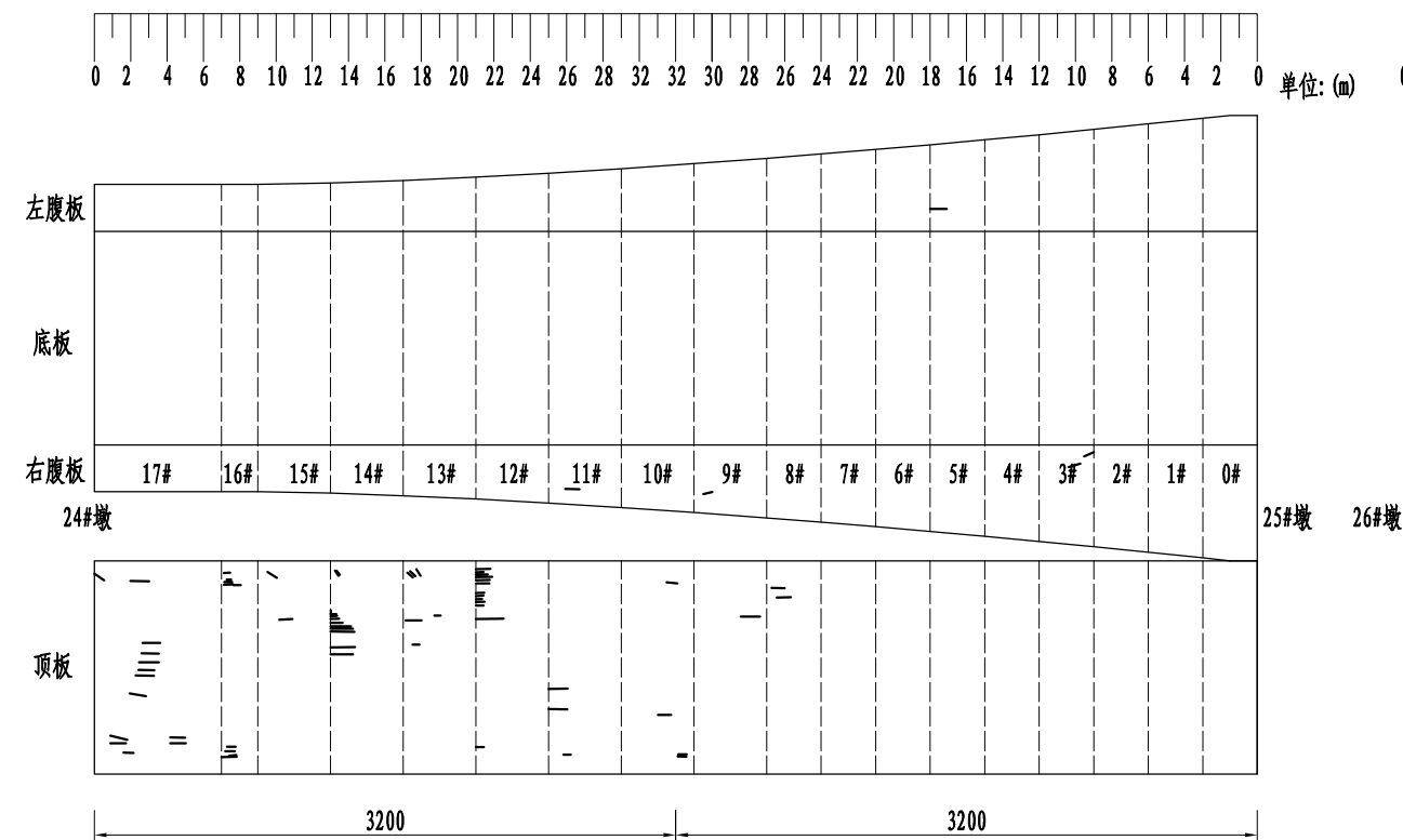
右幅51#孔箱梁内表面病害分布图
