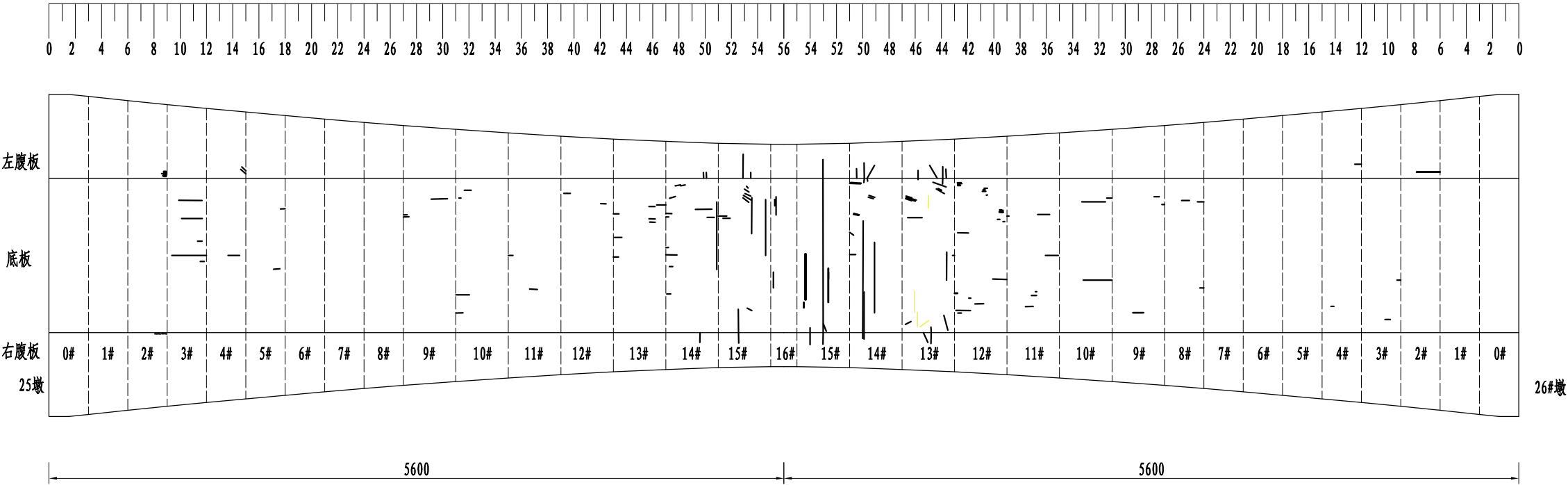
左幅52#孔箱梁外表面病害分布图
