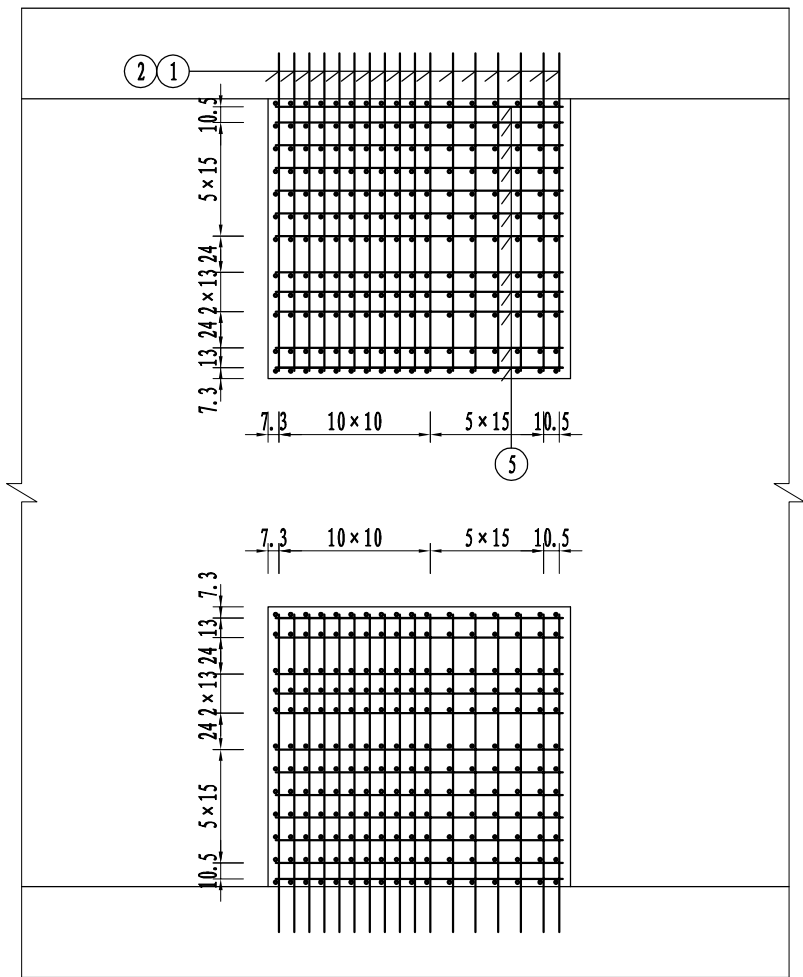
平面
