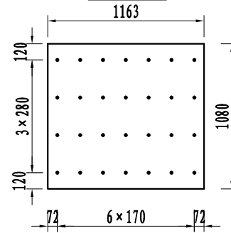
N4钢板
