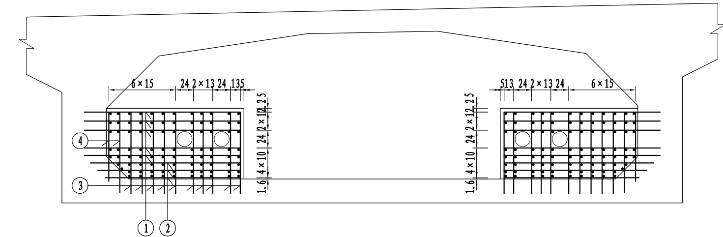
齿板1钢筋数量表
