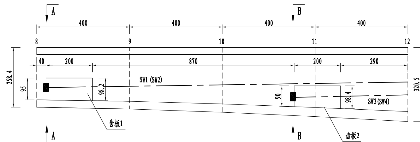
平面图
