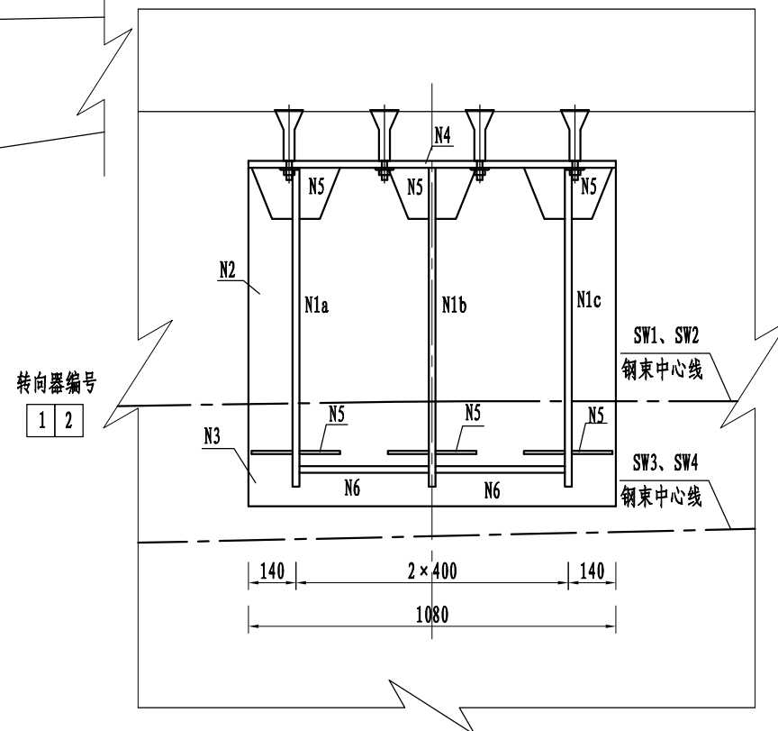
新增转向块1立面图
