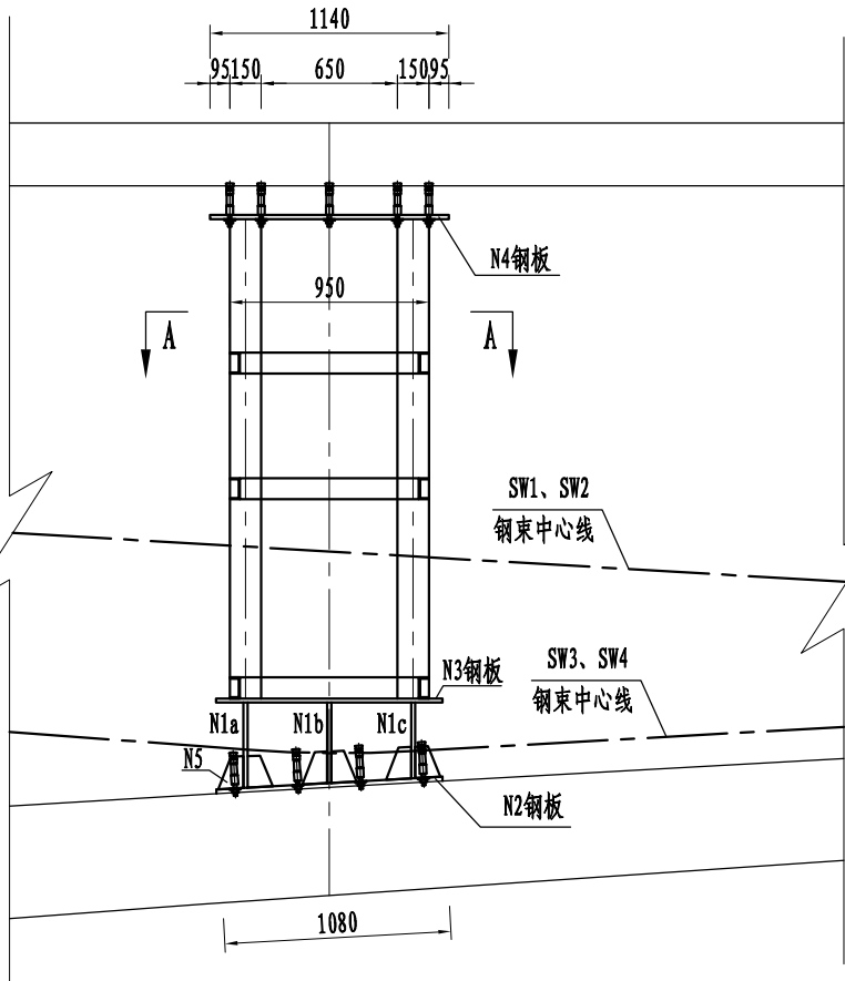
新增转向块5立面图
