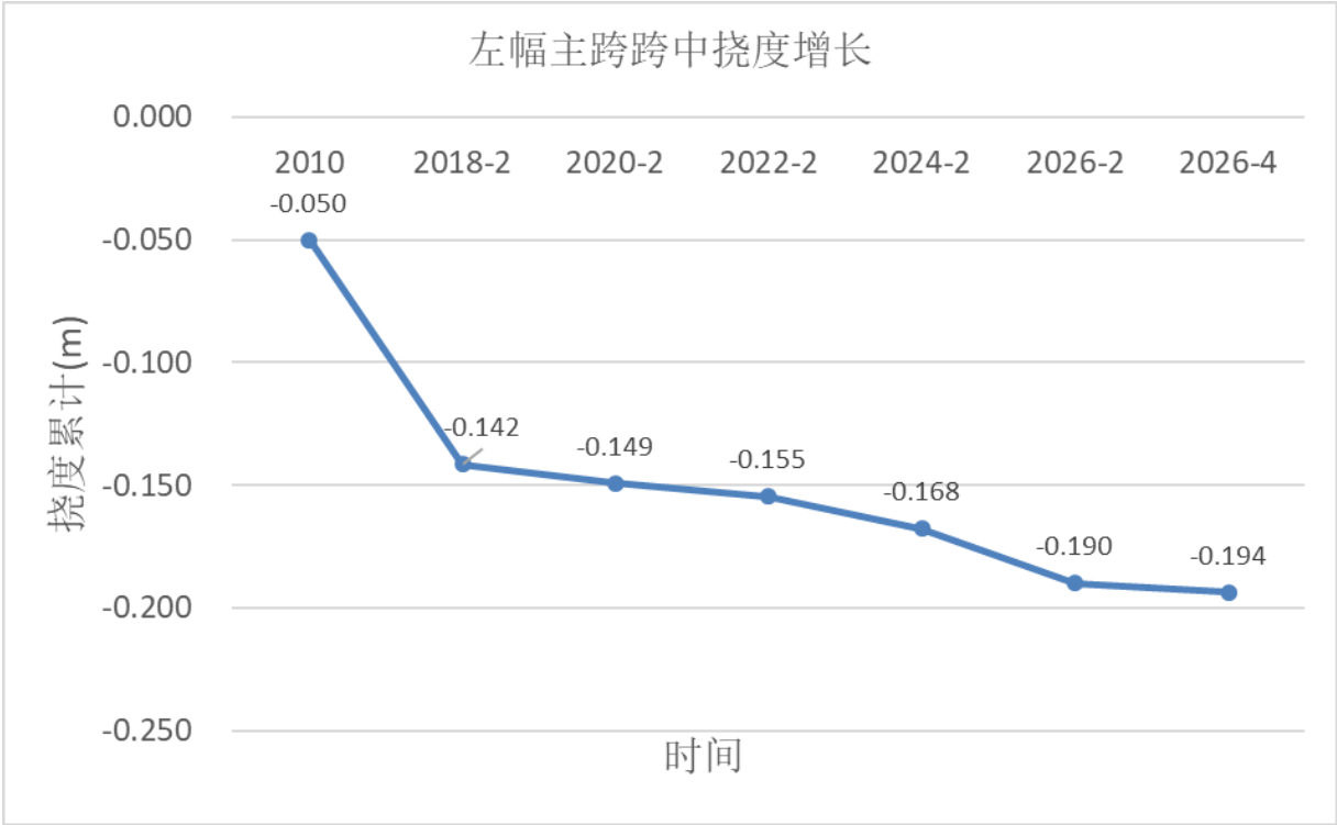
图 2-4 左幅主跨跨中挠度累计增长量（单位：m）
