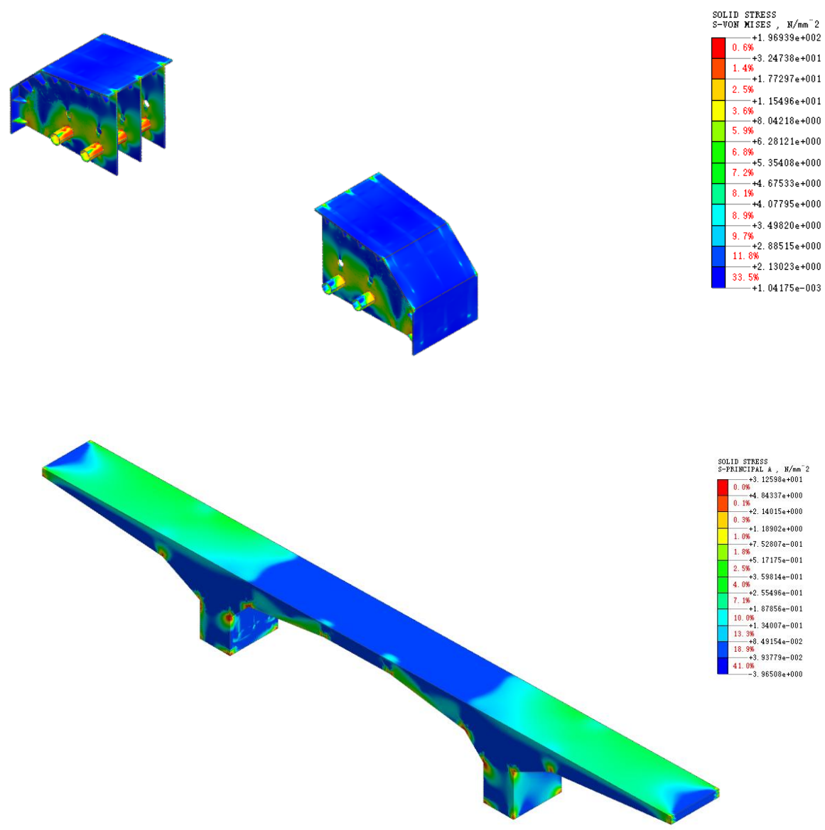
图 6-12 3#钢结构转向块有限元分析
