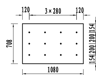
N2钢板
