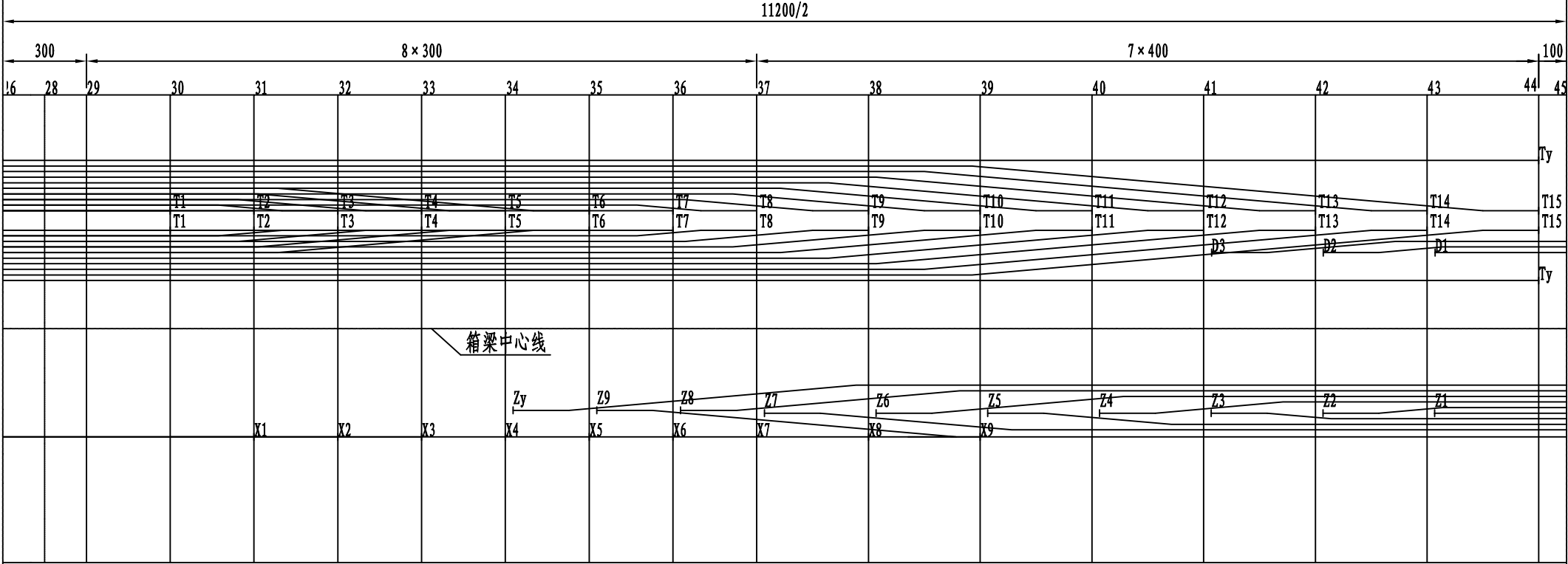
1/2中跨钢束底板半平面布置
