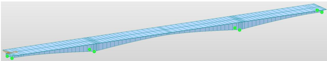
图 3-1 梁单元模型
