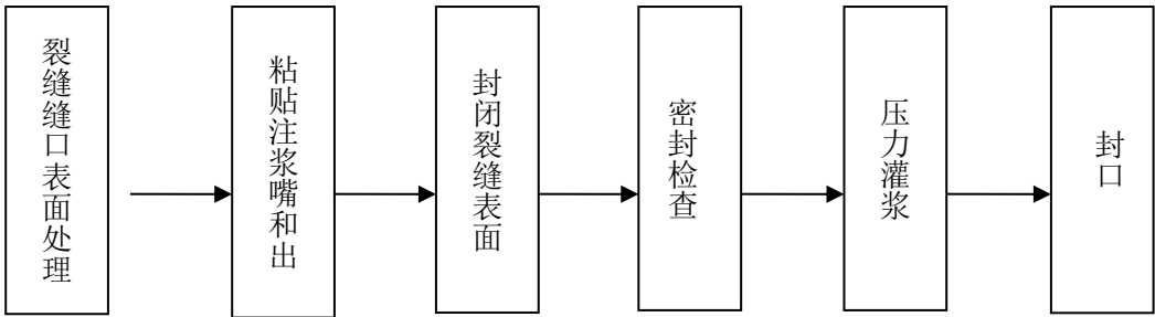
图 7-4 裂缝压力灌浆施工工艺流程
