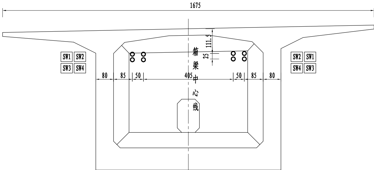
墩顶中横梁开孔横断面图
