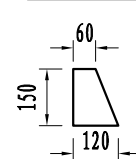
N5钢板
