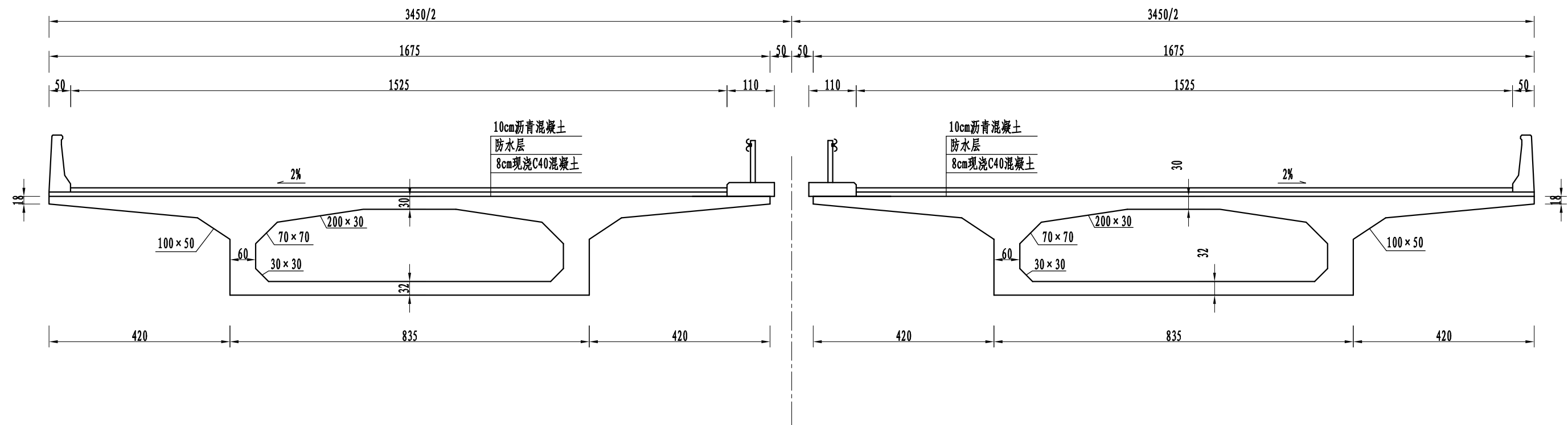
典型横断面
