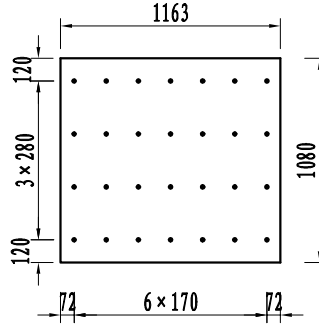
N4钢板
