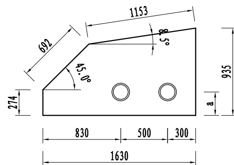
N3钢板
