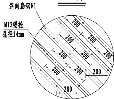
A大样
