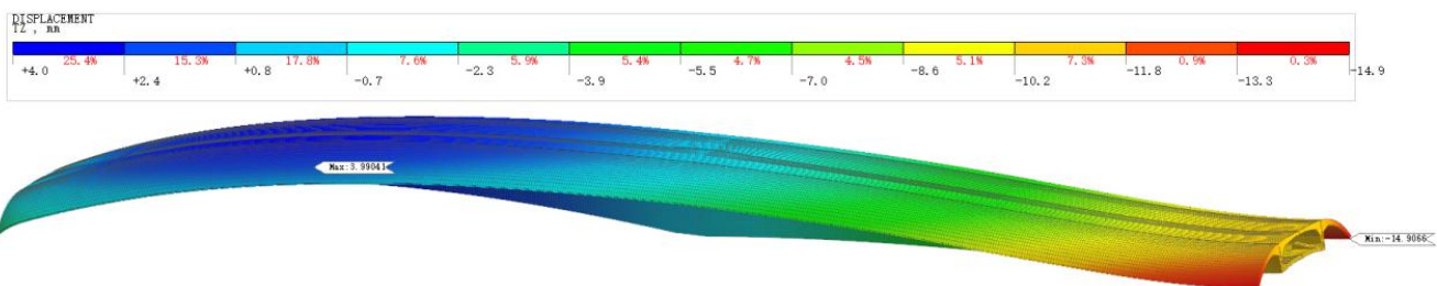
图 4-8 梯度升温作用的横向框架弯曲变形图（mm）
