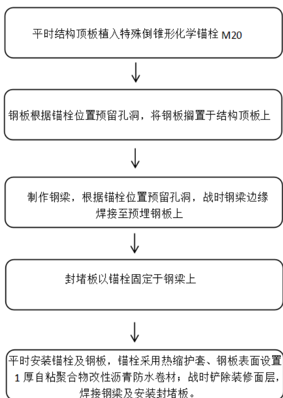
水平封堵构件的安装流程示意图
