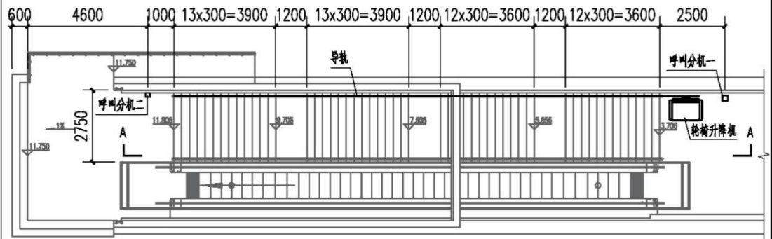
2号出入口轮椅升降机平面布置图
