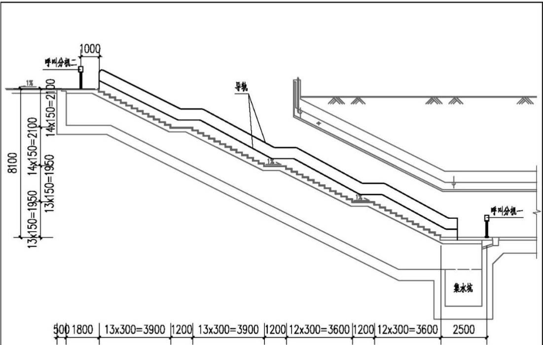
A-A剖面图
