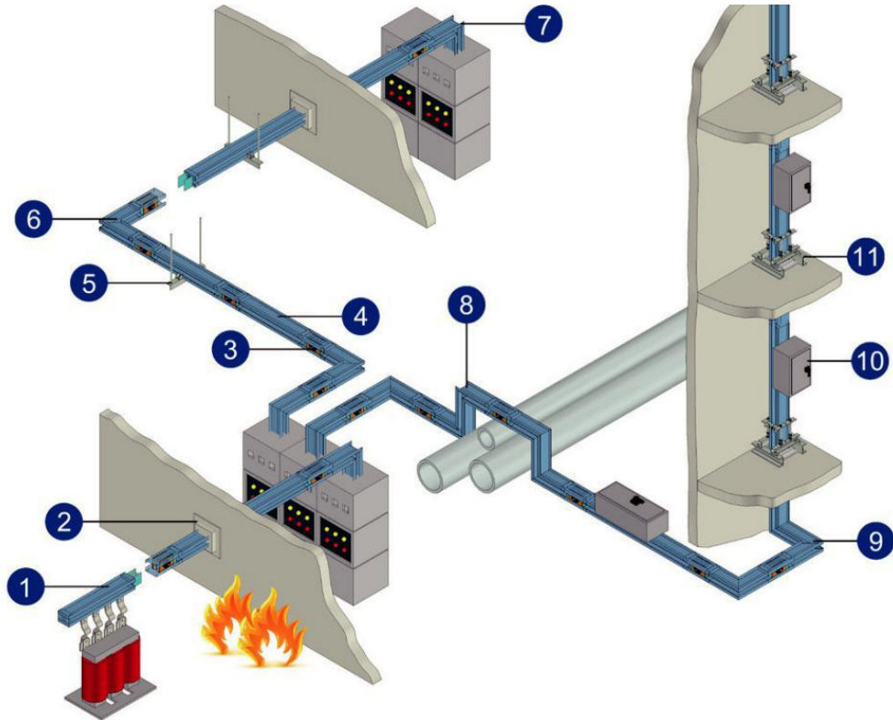
图2.1-1 低压密集型母线槽产品结构组成示意图
