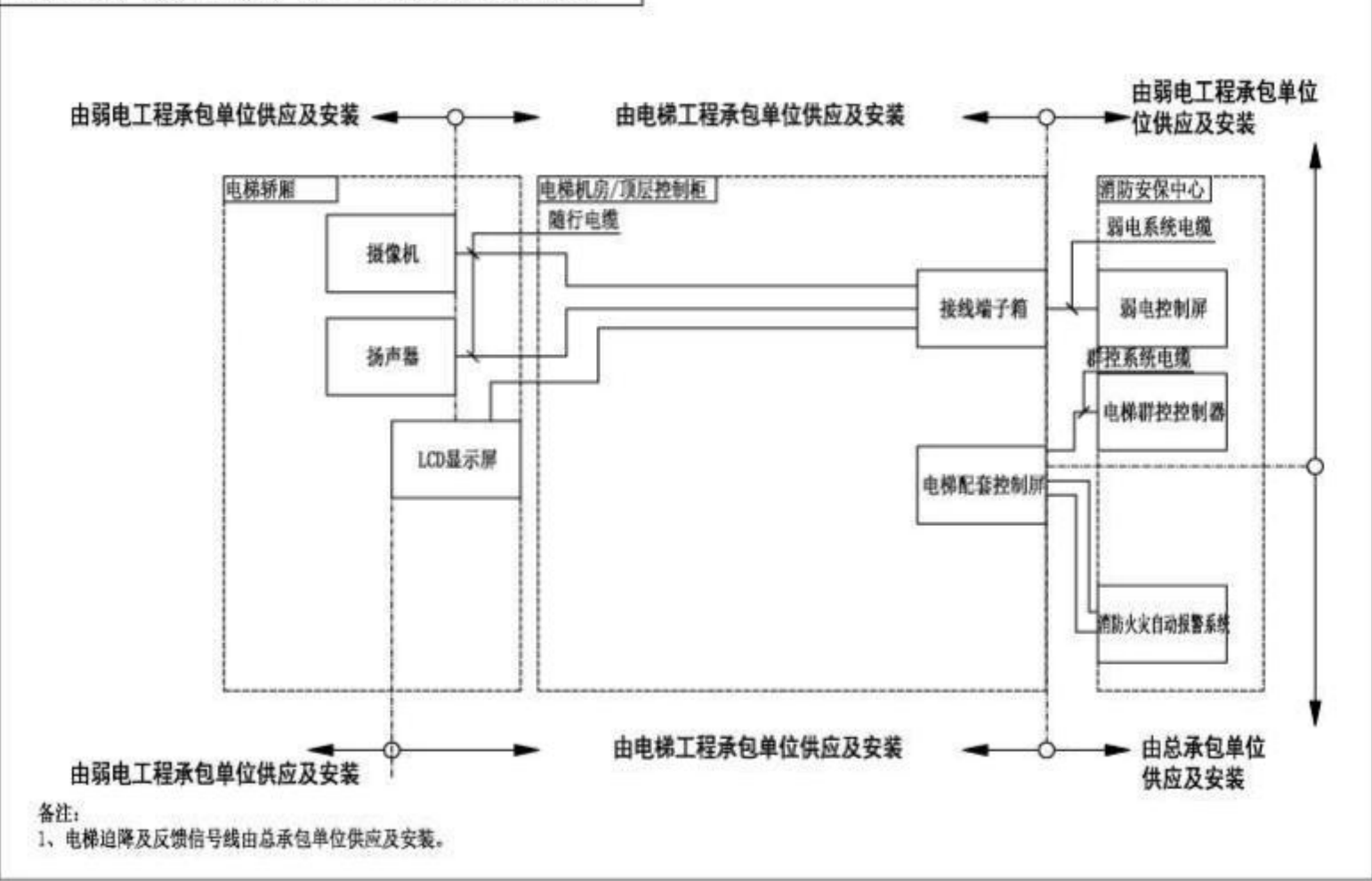
电梯工程（弱电部分）承包单位分界面示意图
