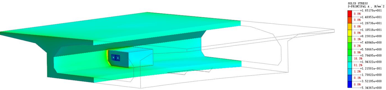
图 6-11 典型齿板有限元分析
