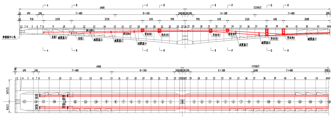
图 5-2 增设钢束方案
