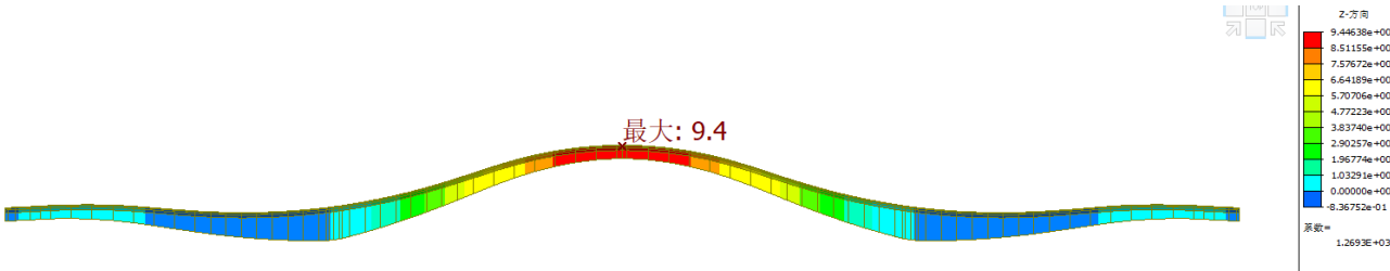
图 6-10 加固后主梁竖向挠度图（mm）
