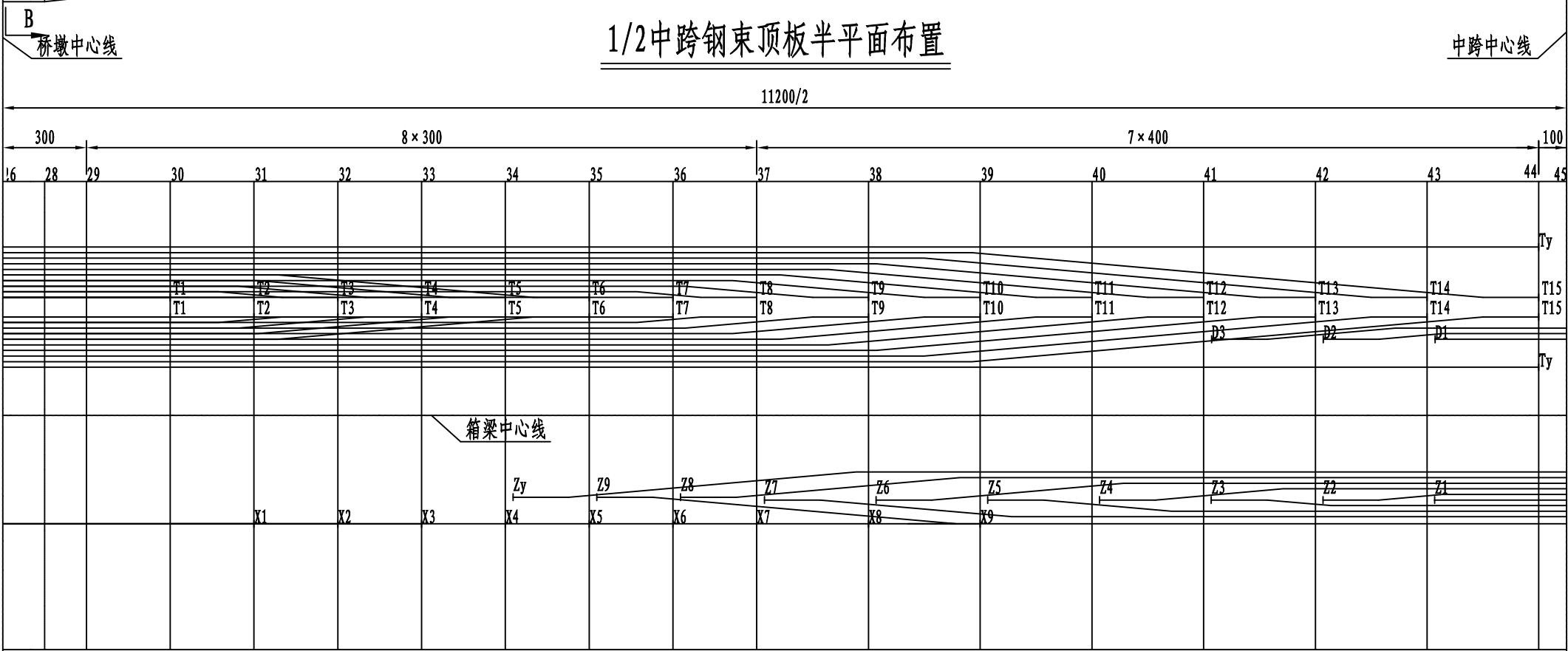
1/2中跨钢束底板半平面布置
