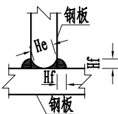
钢板连接大样1
