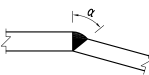
钢板连接大样2
