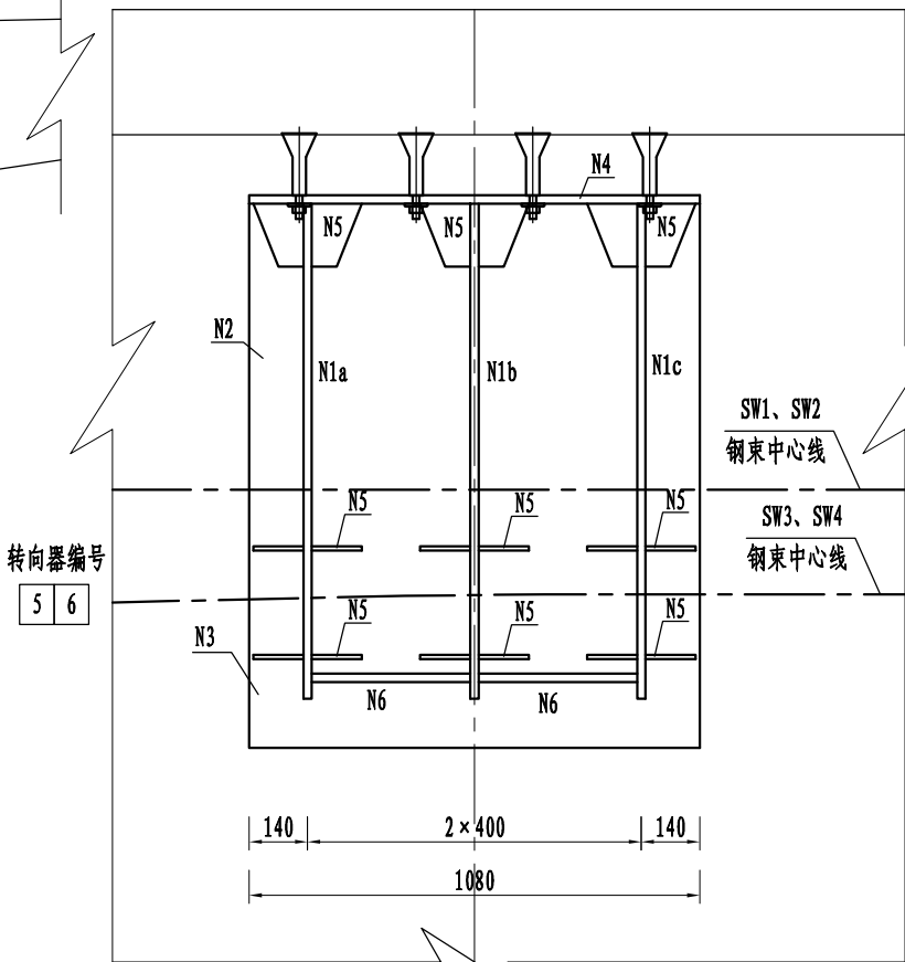
新增转向块3立面图
