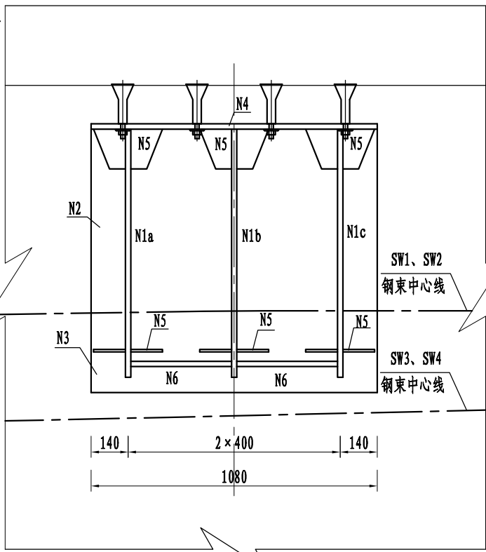
新增转向块1立面图
