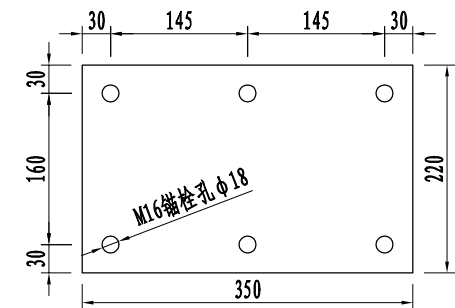
锚固钢板大样
