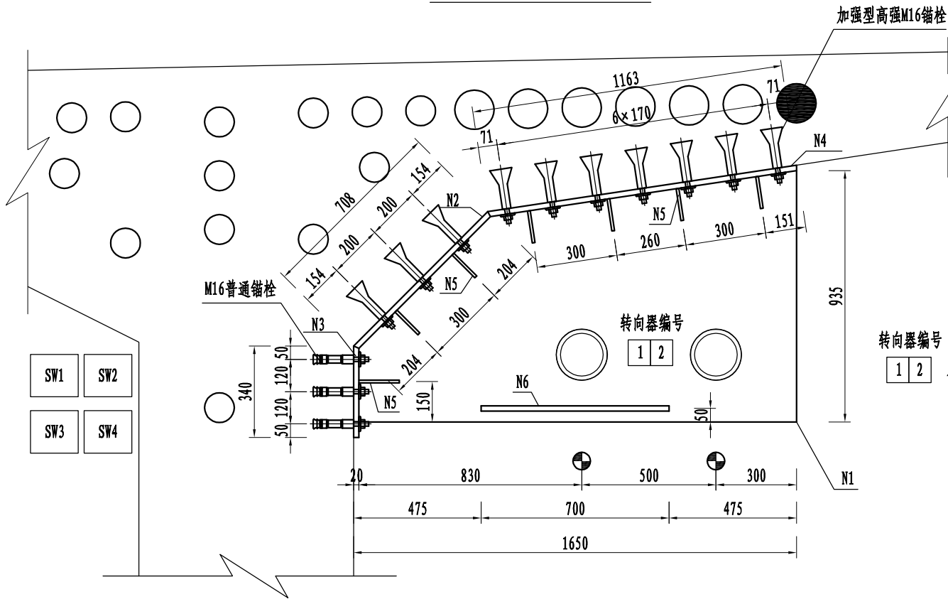
新增转向块1断面图
