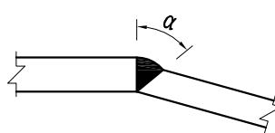
钢板连接大样2
