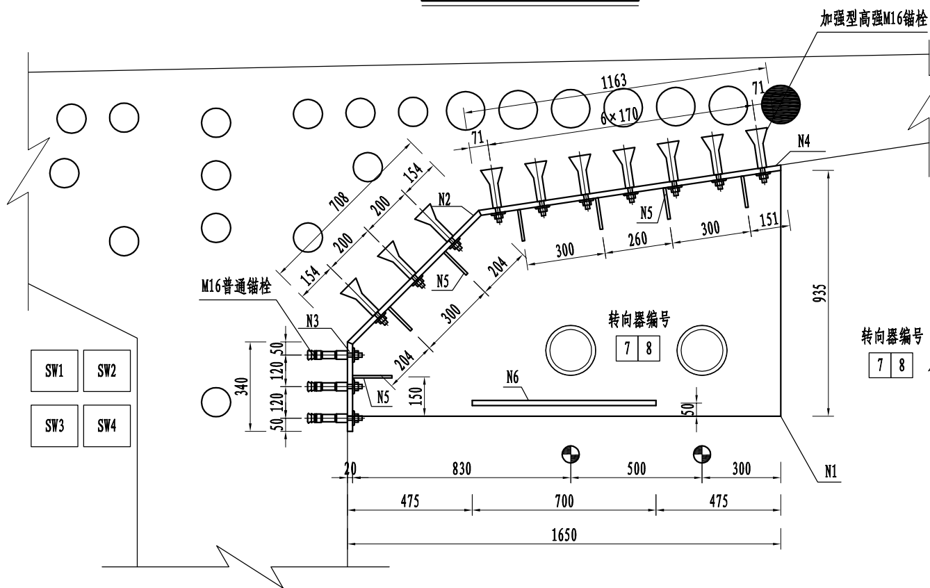
新增转向块4断面图
