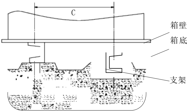
图又 箱底支架焊接位置（长轴方向）
