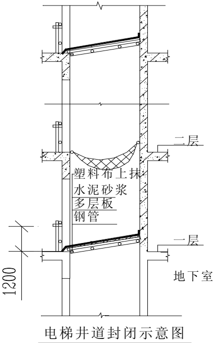
电梯厅井道楼层临时封闭示意图：
