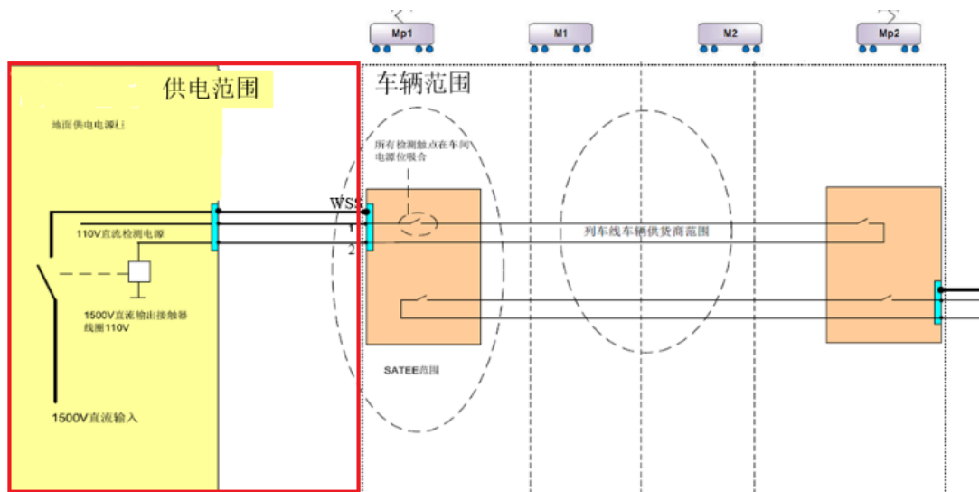
图 2 电气电路示意图
