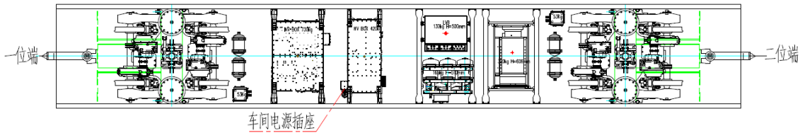
图 1 静调电源插座布置图
