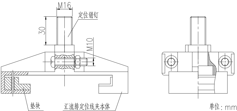
B 型汇流排定位线夹（仅为示意）
