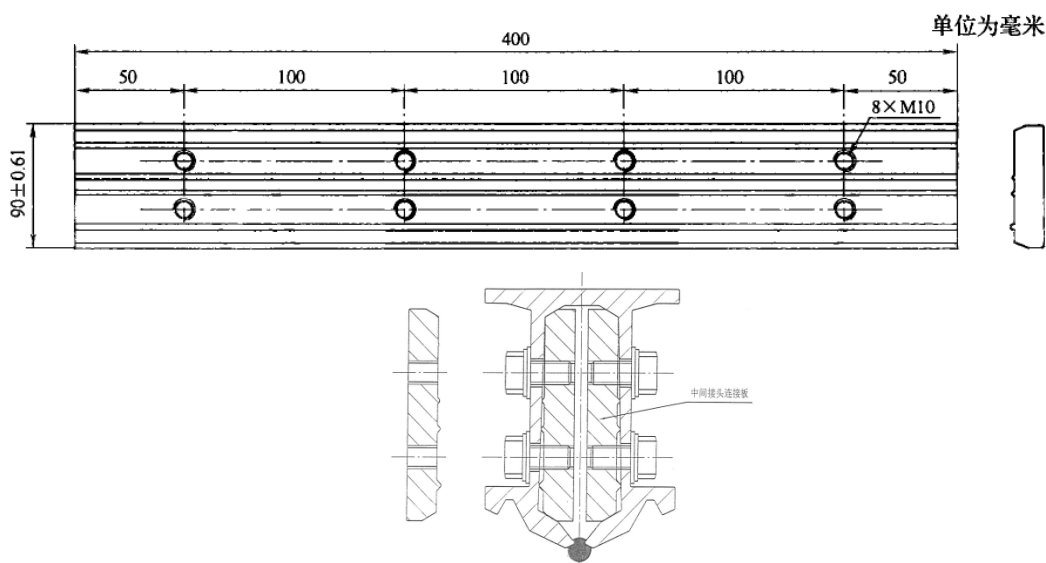
图 2 汇流排中间接头外形及尺寸示意图
