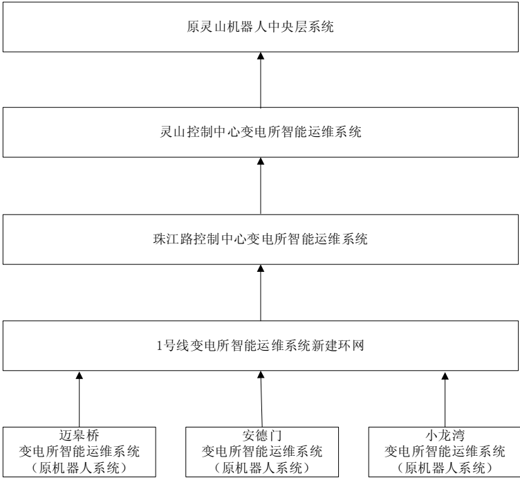
此图仅做本次变电所智能运维系统与既有南京地铁供电主所智能机器人系统融合通讯示意图
