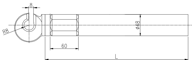
48 型定位管
