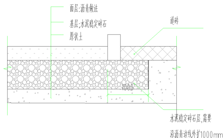
道路剖面节点图
