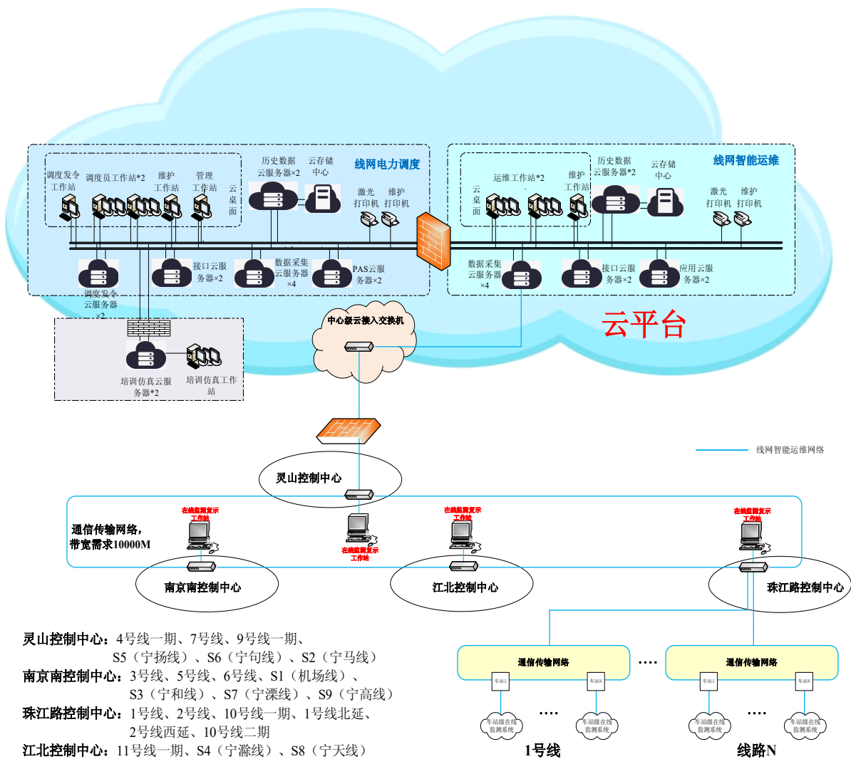
线网智能运维系统网络架构
