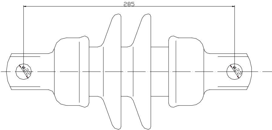
图 1 瓷质下锚绝缘子（尺寸：mm）
