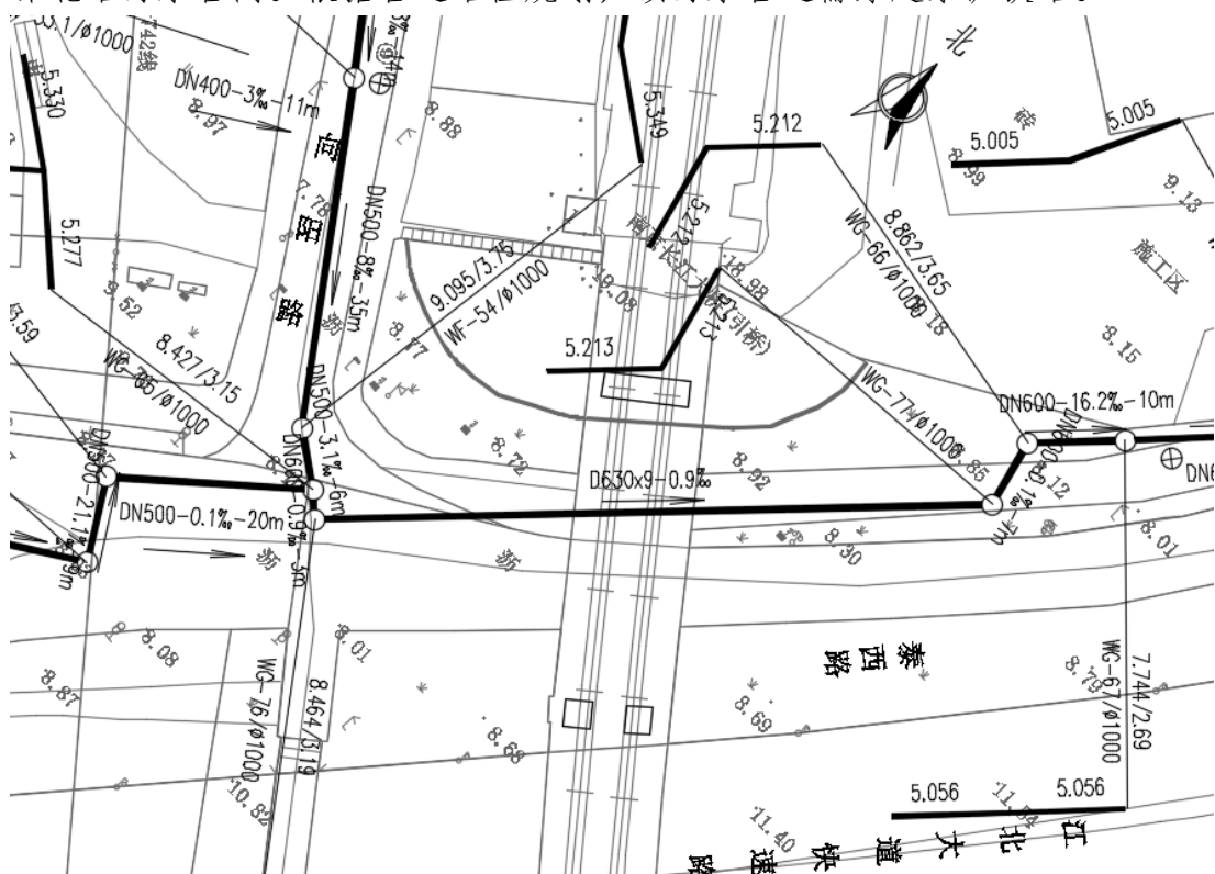
图 1 污水管线路平面图
