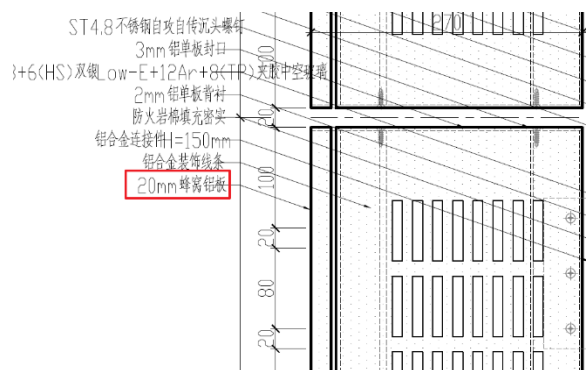
节点图 C-T-5303
