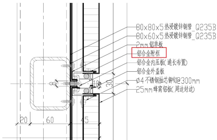
节点图 C-T-5207
