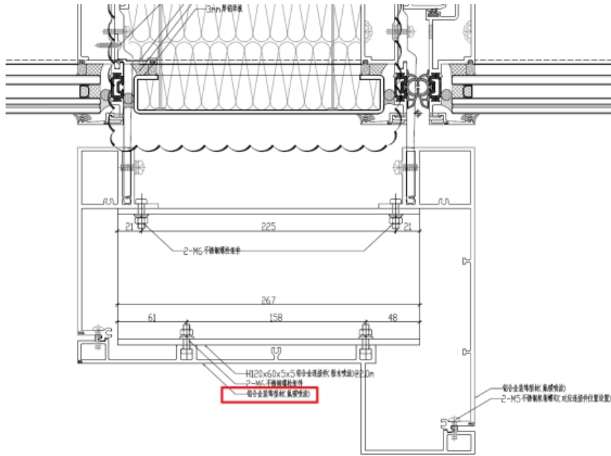
节点图 C-T-5101
