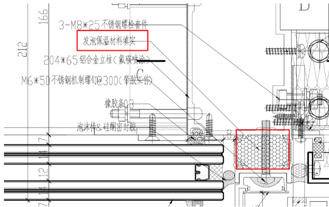
节点图 C-S-5101
