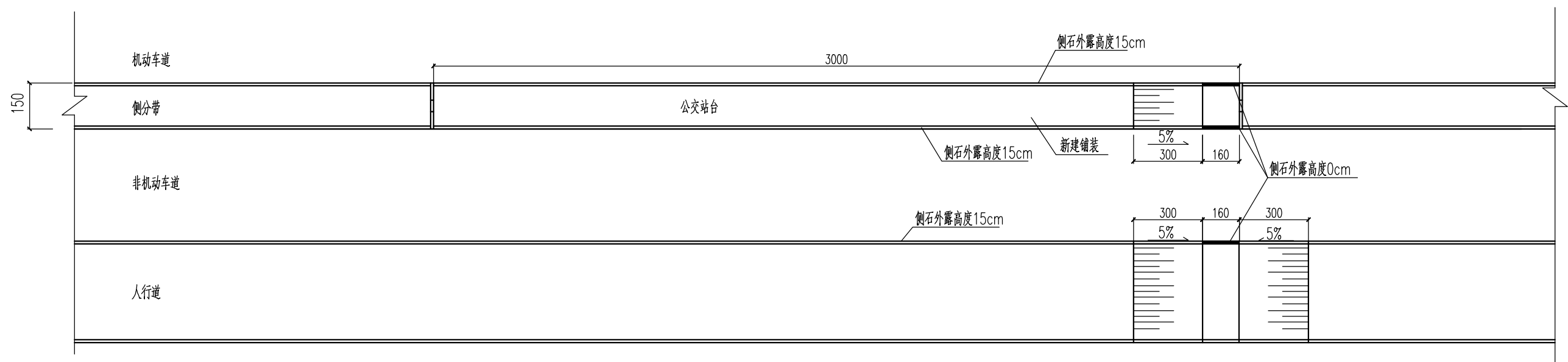
公交站台处缘石坡道平面图 1:200
