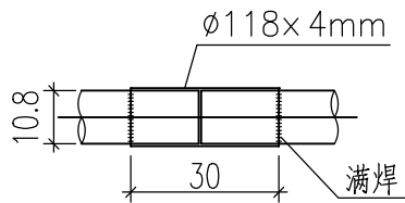
钢管对接图
