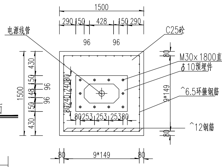
基础配筋平面
