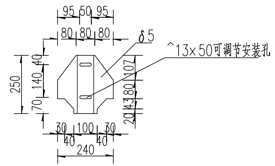
横臂法兰
