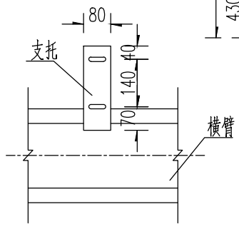
计数屏支托正立面
