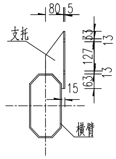
计数屏支托侧立面
