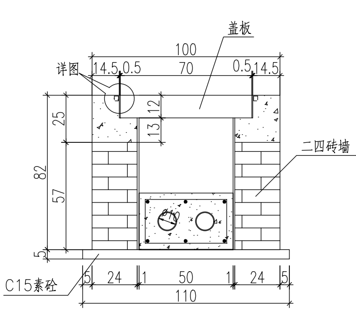
A—A 1:20
