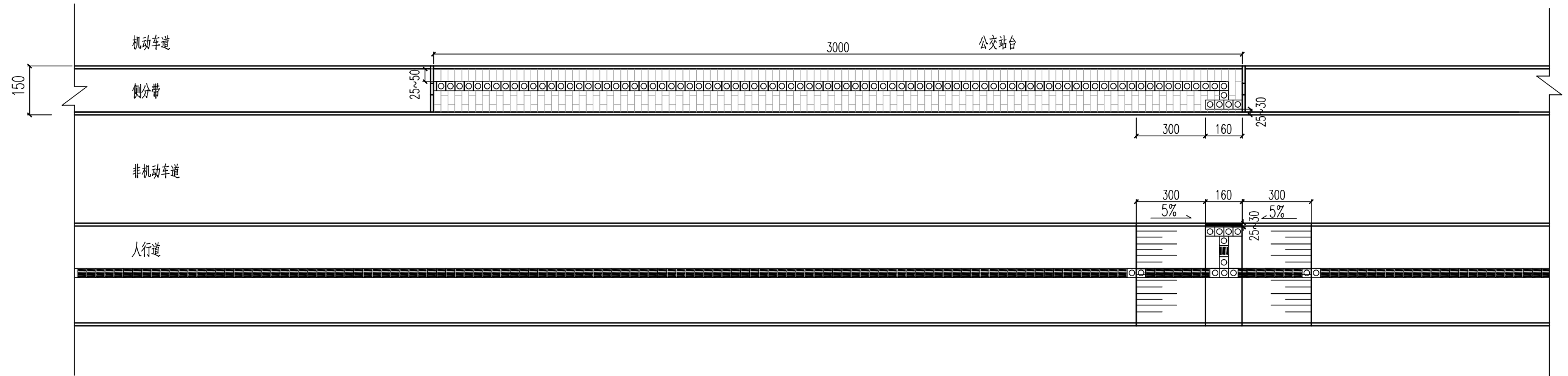
公交站台处盲道布置大样图 1:200
