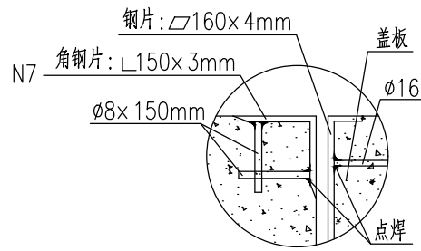
详图
