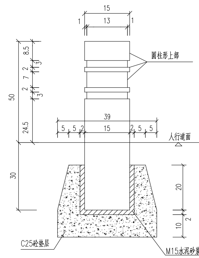
花岗岩阻车石构造大样图
