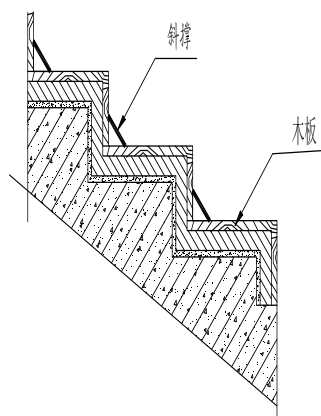
地砖楼梯踏步保护
