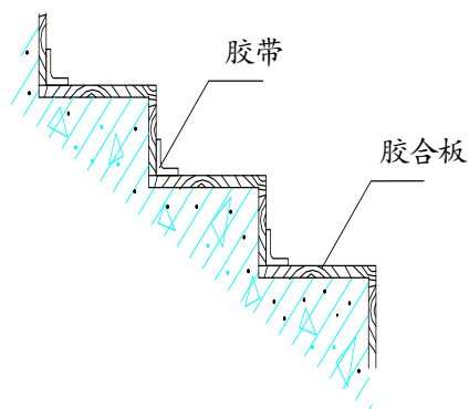
抹灰完成后的楼梯踏步保护
