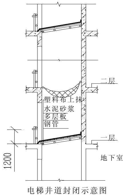
电梯厅井道楼层临时封闭示意图：
