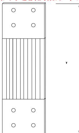
图1 变压器与低压柜或低压柜间连接段槽形母线长度计算（图片仅供参考）
