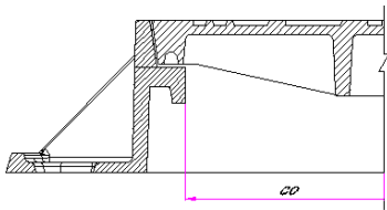
球铁井框盖局部剖面
