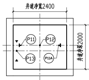
底坑受力图
