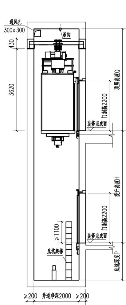
A-A剖面图
