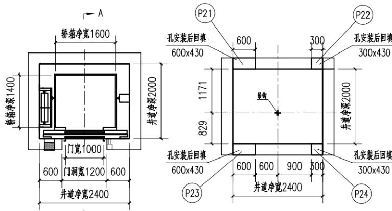
井道顶部吊钩位置图
