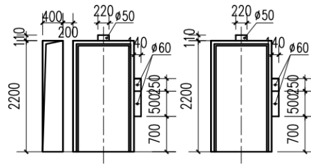
顶层门洞 (从井道外侧看)
